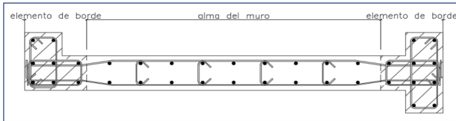
Figura 10. Ejemplo de elementos de borde en muros, Norma E 060 de Concreto Armado, 2019.
