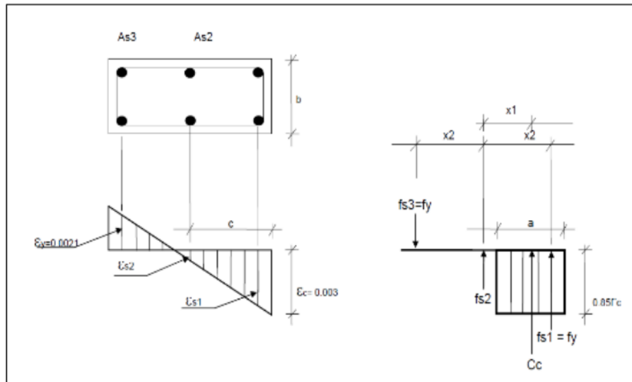
Figura 20. Estado de equilibrio para condición balanceada. Blanco A.
