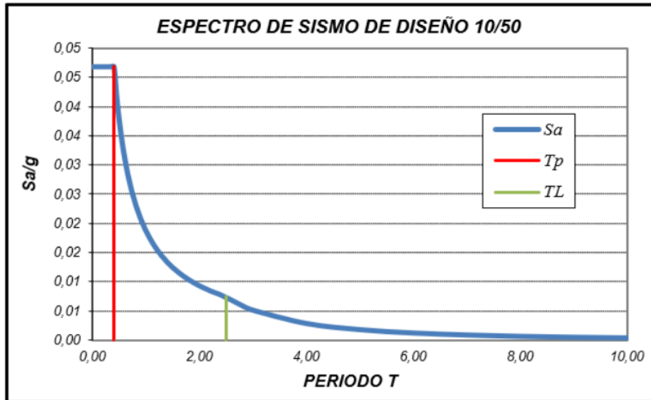
Figura 14. Espectro de diseño, Elaboración propia
