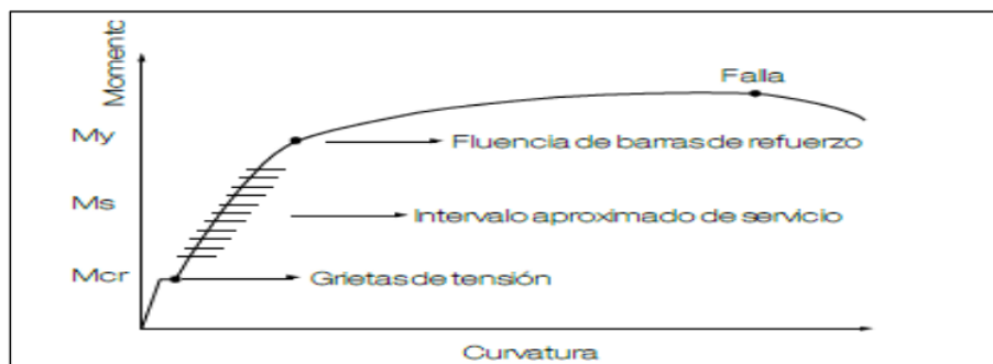
Figura 18. Diagrama de Momento - Curvatura
