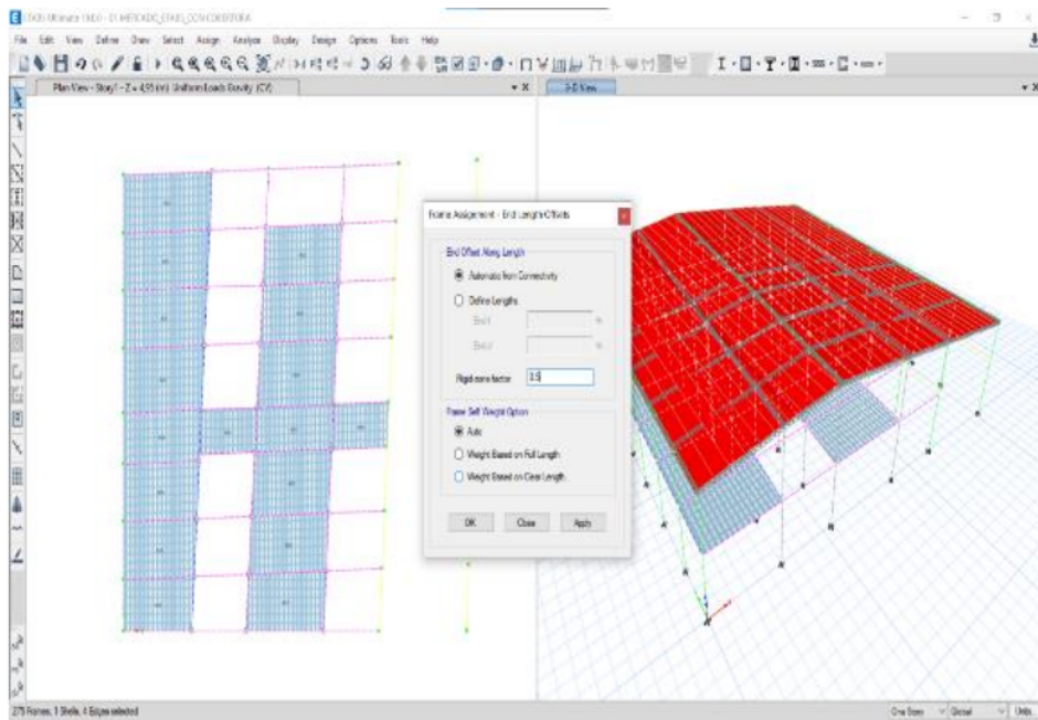
Figura 45. Asignación de brazos rígidos a los pórticos, elaboración propia ETAPS V19
