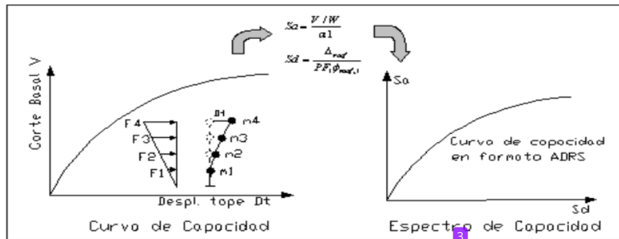
Figura 21. Procedimiento para obtener el espectro de capacidad, Lucio Fernando Sánchez Sarmiento, Pablo Enrique Caiza Sánchez, Ing.M.Sc.
