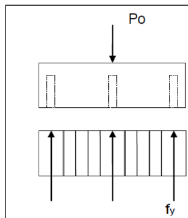
Figura 19. Estado de equilibrio en compresión pura. Blanco A.
