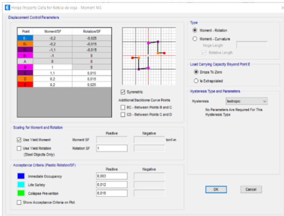
Figura 70. Comportamiento de rotulas manuales en vigas
