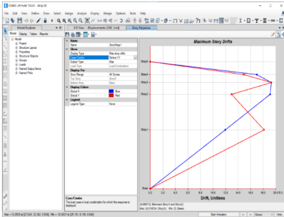
Figura 50. Verificación de derivas y desplazamiento en Y. elaboración propia ETAPS V19
