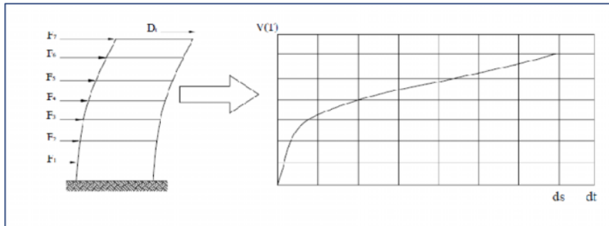
Figura 66. Esquema de la Técnica del Pushover
