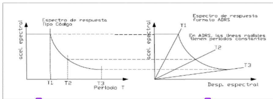
Figura 22. Espectro de respuesta tipo código y en formato ADRS, Lucio Fernando Sánchez Sarmiento, Pablo Enrique Caiza Sánchez, Ing.M.Sc.
