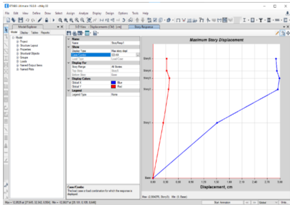
Figura 49. Verificación de derivas y desplazamiento en X, elaboración propia ETAPS V19
