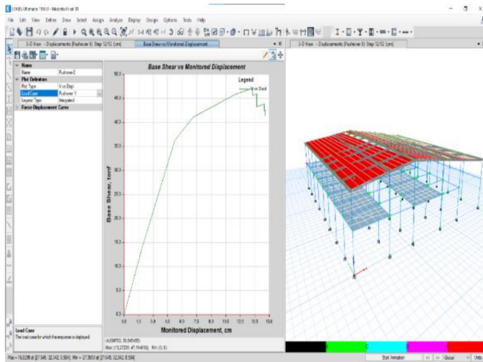
Figura 52. Curva Pushover en Y
