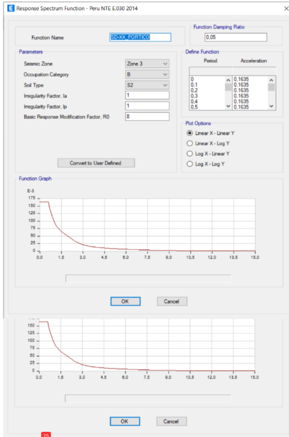
25 Figura 38. Espectro de respuesta en direcciones X y Y, elaboración propia ETAPS V19.
