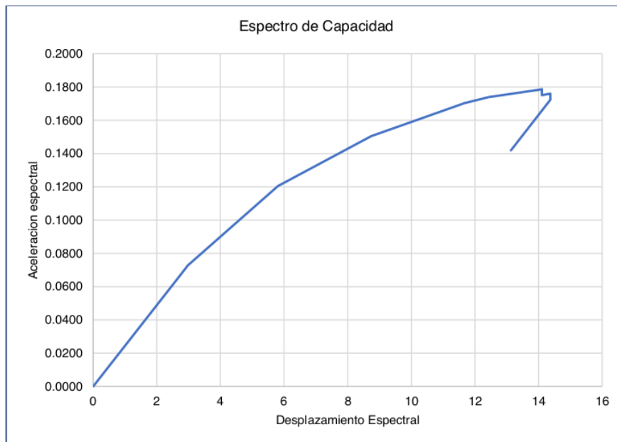
Figura 55. Curva de Capacidad en el sentido X.
