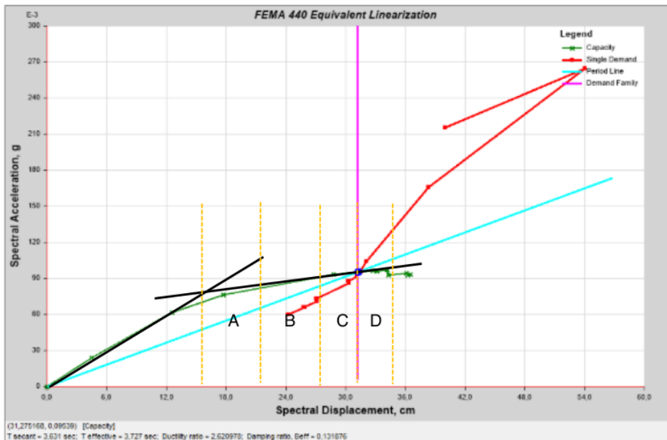
Figura 61. Parametrización de la Curva Pushover en Y
