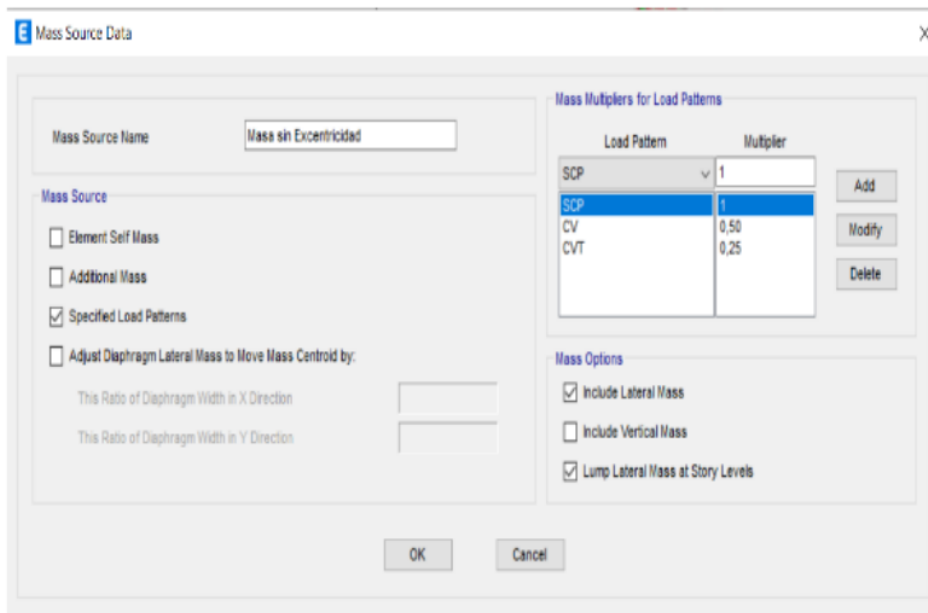
Figura 77. Definición de masa sin excentricidad
