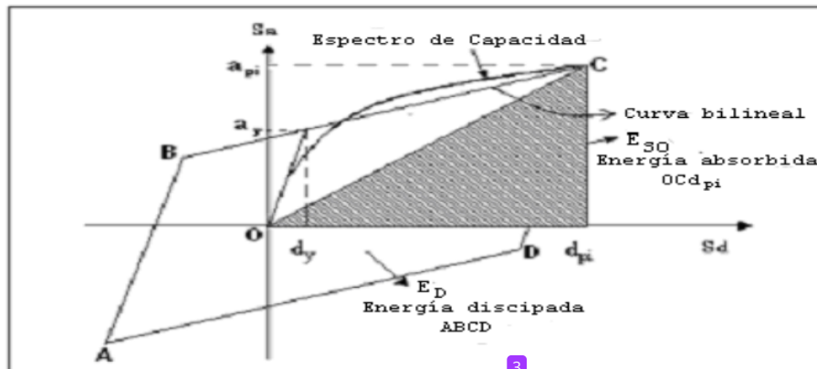
Figura 24. Espectro de capacidad, punto de desempeño, Lucio Fernando Sánchez Sarmiento, Pablo Enrique Caiza Sánchez, Ing.M.Sc.
