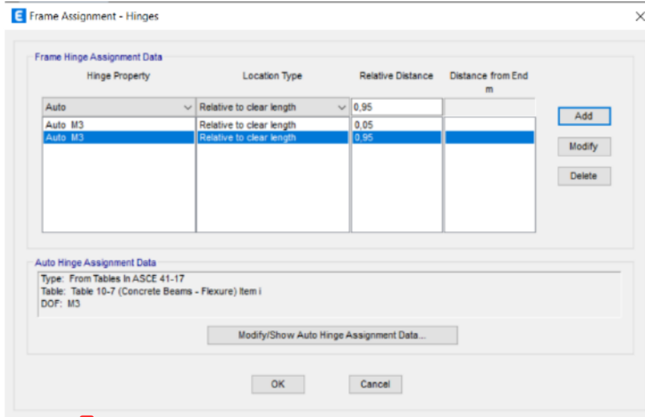
Figura 69. Asignación de rotulas automáticas en vigas
