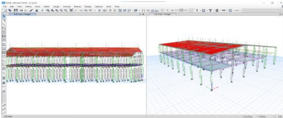
Figura 73. Rotulas en vigas y columnas en 3D
