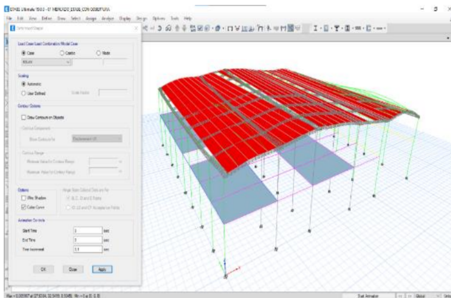
Figura 48. Análisis de resultados, elaboración propia ETAPS V19
