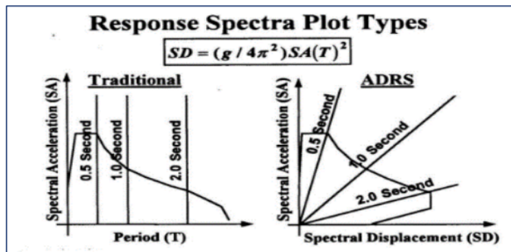
Figura 9. Diagrama de tipos de respuesta espectral, Freeman 1998
