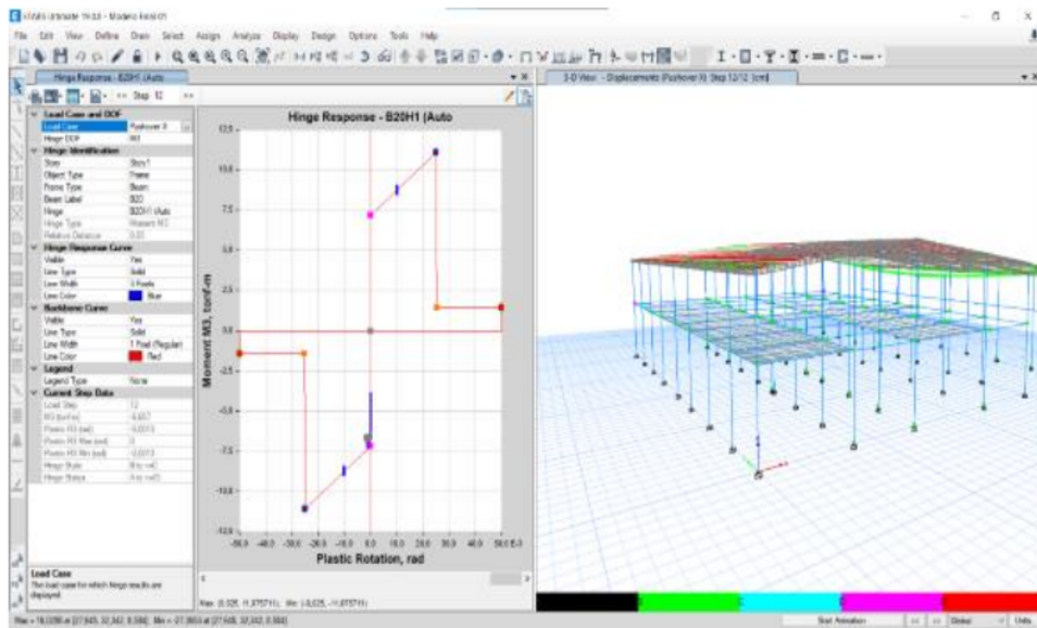
Figura 53. Análisis de la viga B20H1
