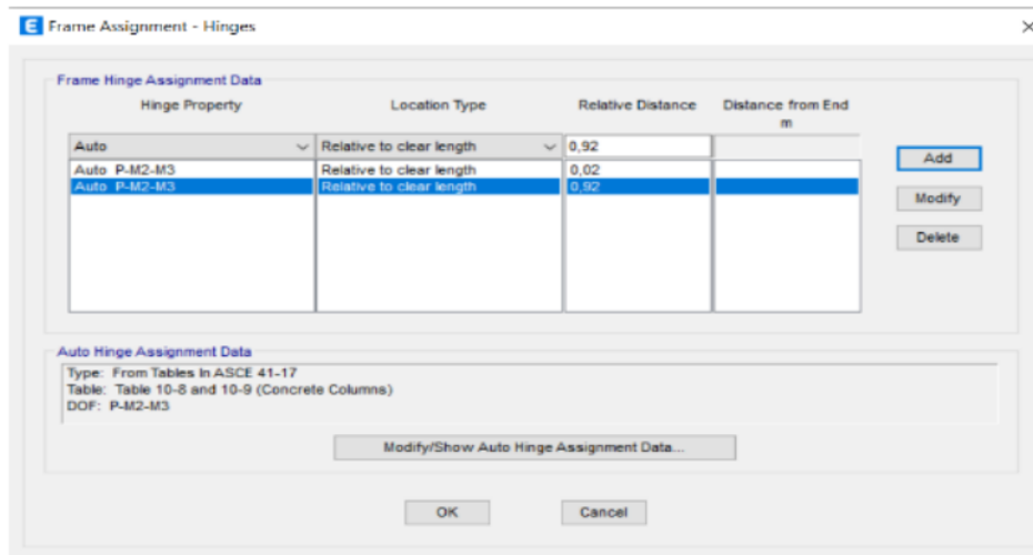
Figura 72. Creación de rotulas en columnas
