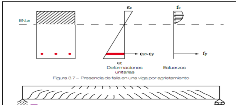
Figura 17. Viga con falla de agrietamiento.
