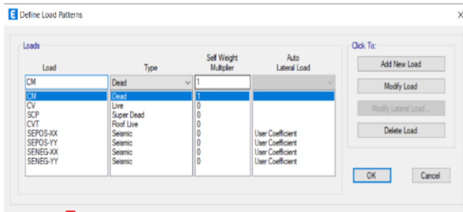
1 Figura 37. Casos de carga, elaboración propia ETABS V19.
