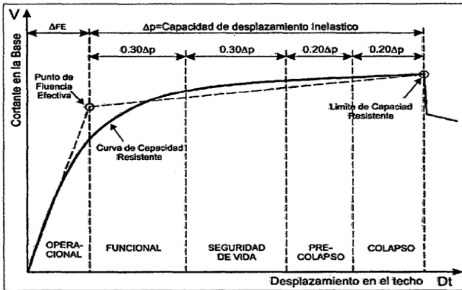
Figura 60. Rango de parámetros de la curva Pushover.
