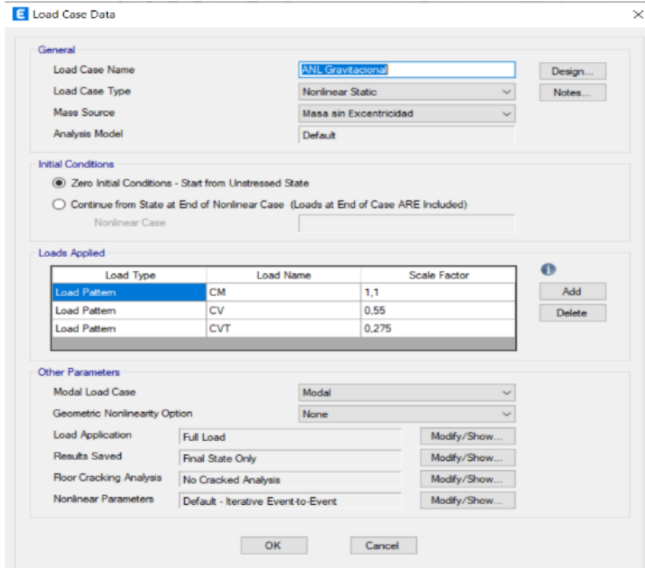
Figura 78. Creación de caso de carga según FEMA 356 artículo 3.2.8
