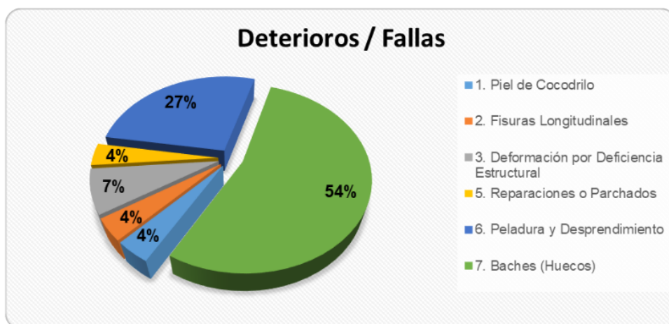
Figura 32. Deterioros / Fallas identificadas del tramo en estudio
