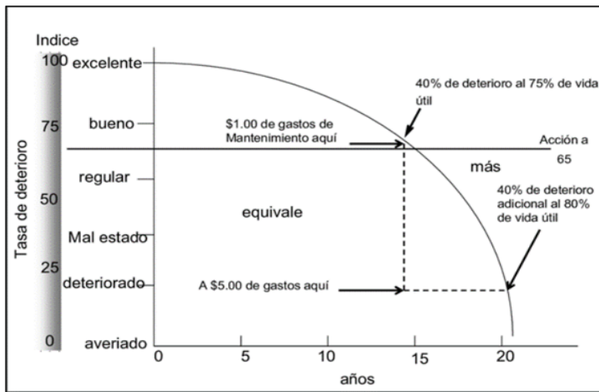
Figura 1. Curva de comportamiento de los pavimentos Fuente: Delmar Salomón 2006.
