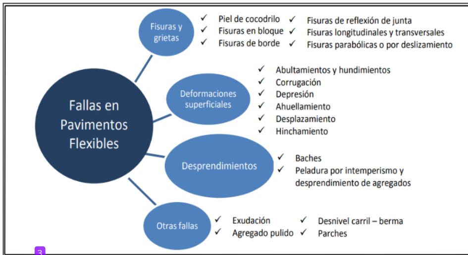
Figura 2. Fallas en pavimentos flexibles
