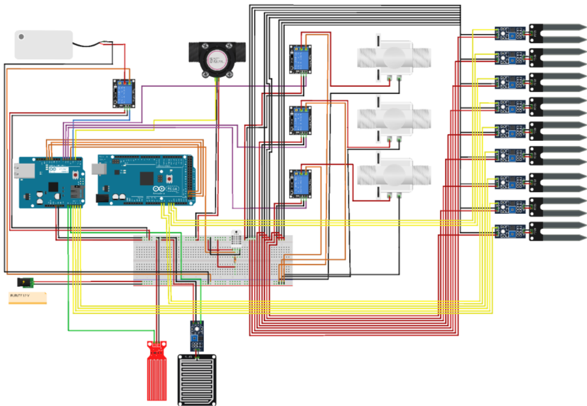
Figura 10. Esquema eléctrico del sistema de riego automatizado
