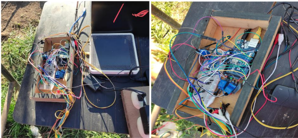
Figura 11. Fotografías del microcontrolador, componente principal del sistema
