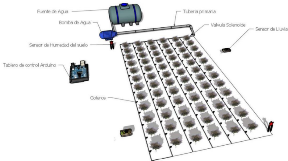
Figura 1. Arquitectura del sistema de riego automatizado por goteos
