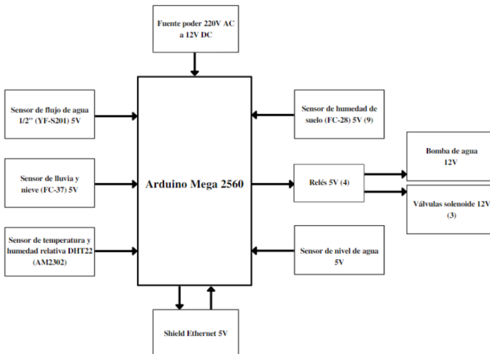
Figura 9. Dispositivos vinculados al microcontrolador
