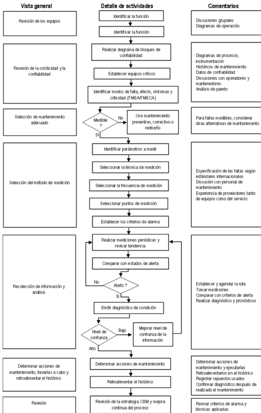
Figura 2. Procedimiento de monitoreo de condición
