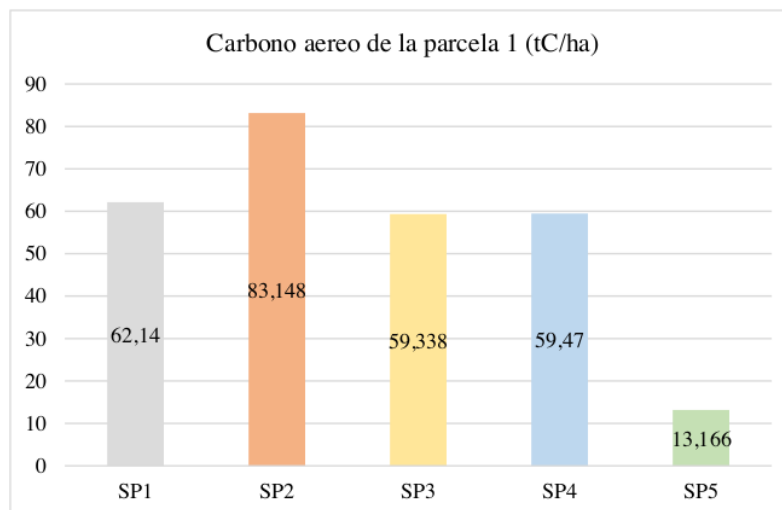
Figura 7. distribución del stock del carbono en (tC/ha) por cada sub parcela de la parcela 1.
