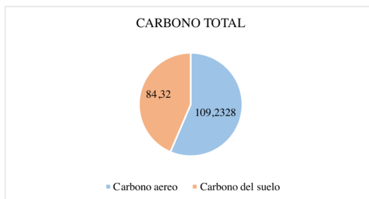
Figura 11. Distribución del carbono total del Eucalyptus torelliana por componente
