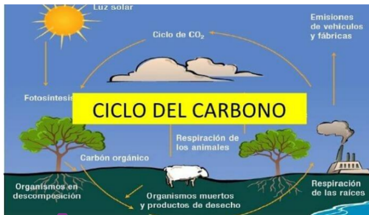
Figura 1. Ciclo del carbono
