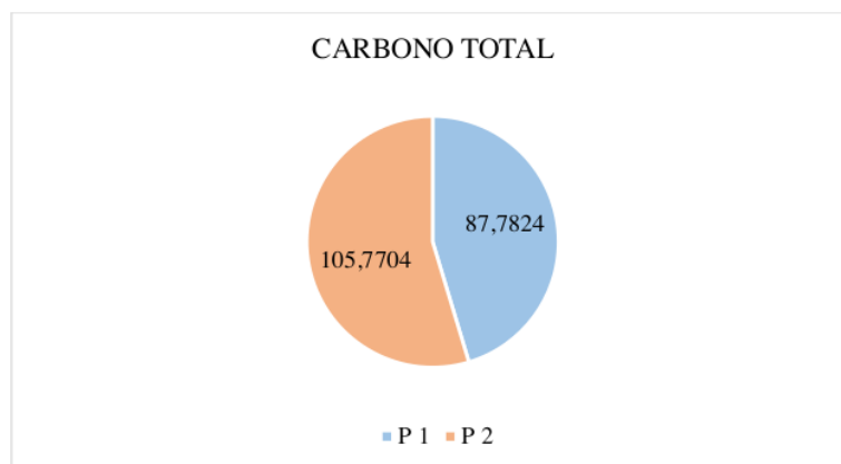
Figura 10. Distribución del carbono total del Eucalyptus torelliana por parcela
