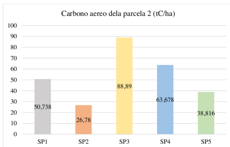
Figura 8. distribución del stock del carbono en (tC/ha) por cada sub parcela de la parcela 2.
