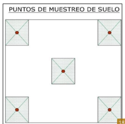
Figura 6. Puntos de muestreo de suelo. Fuente: elaboración propia, basada en la “guía para la determinación de carbono en pequeñas propiedades rurales” (ICRAF, 2009)
