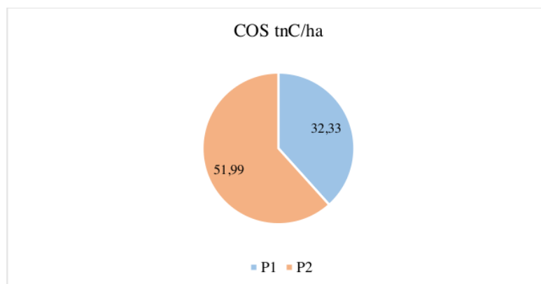
Figura 9. Distribución del carbono en el suelo de la parcela 1 y 2.
