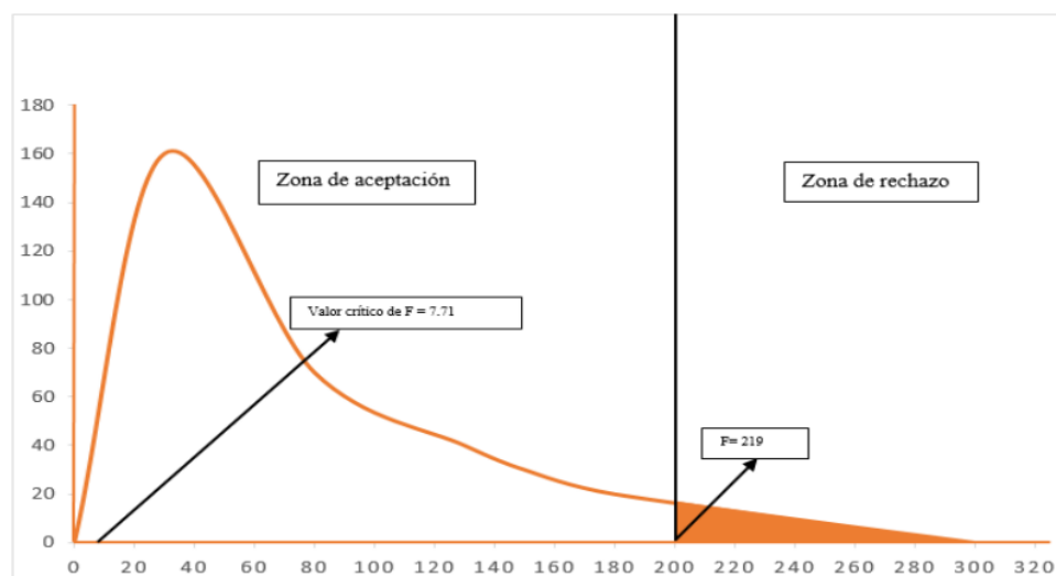
Figura 17. Representación del análisis de varianza
