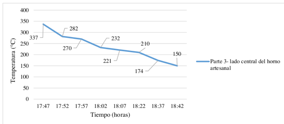
Figura 16. Gráfico de la temperatura durante el horneado
