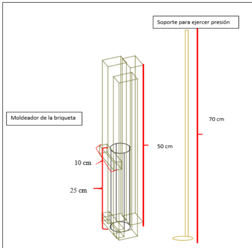
Figura 1. Diseño de la prensa artesanal
