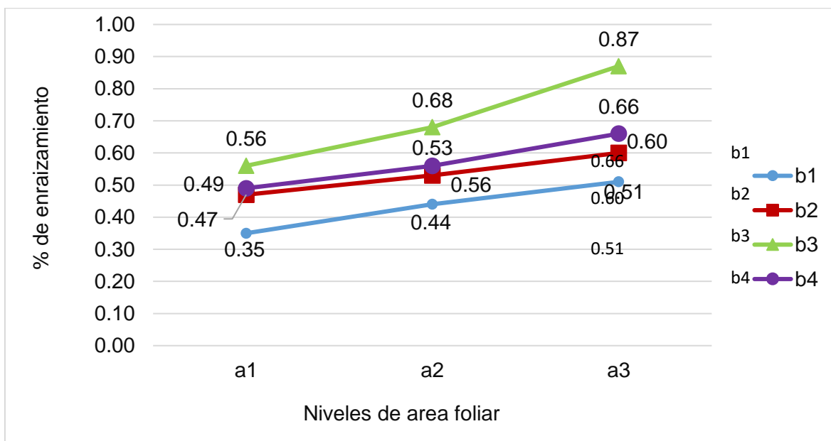
Figura 5. Evaluación del efecto conjunto de la longitud de estacas (Factor A) en los promedios de los niveles del factor B (Área foliar) en el porcentaje de enraizamiento
