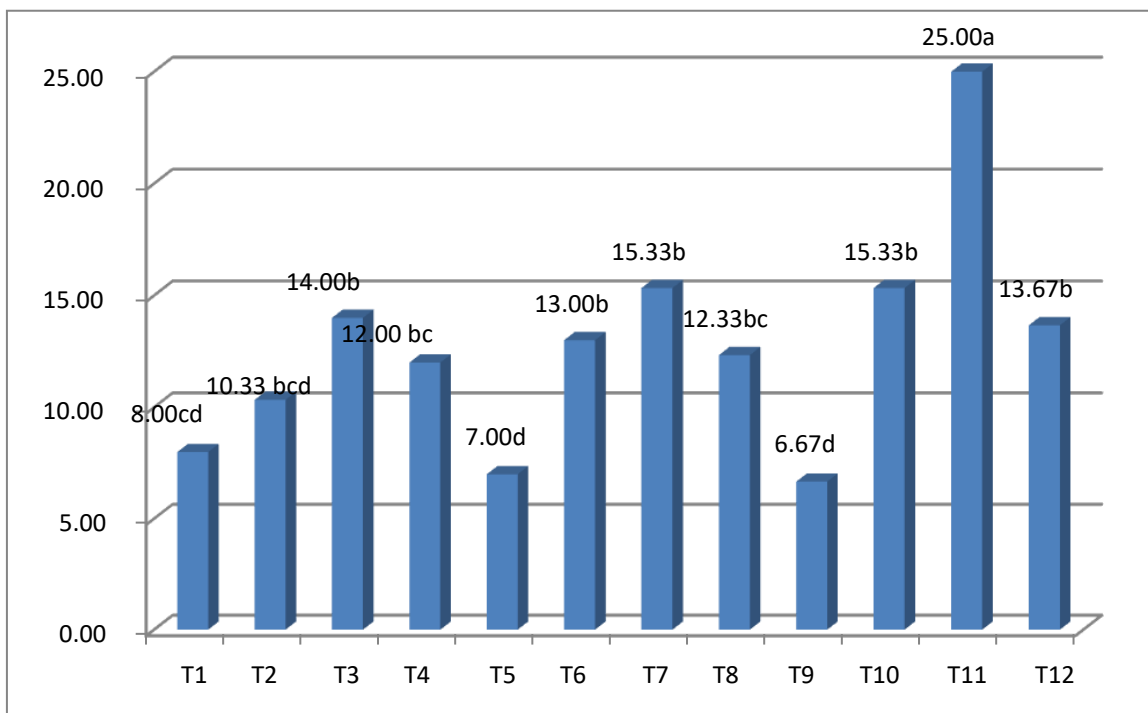
Figura 8. Comparación de los efectos de los factores A y B en el número de raíces mediante la Prueba de Tukey ( \alpha=0.05 ) en diferentes tratamientos raíces.
