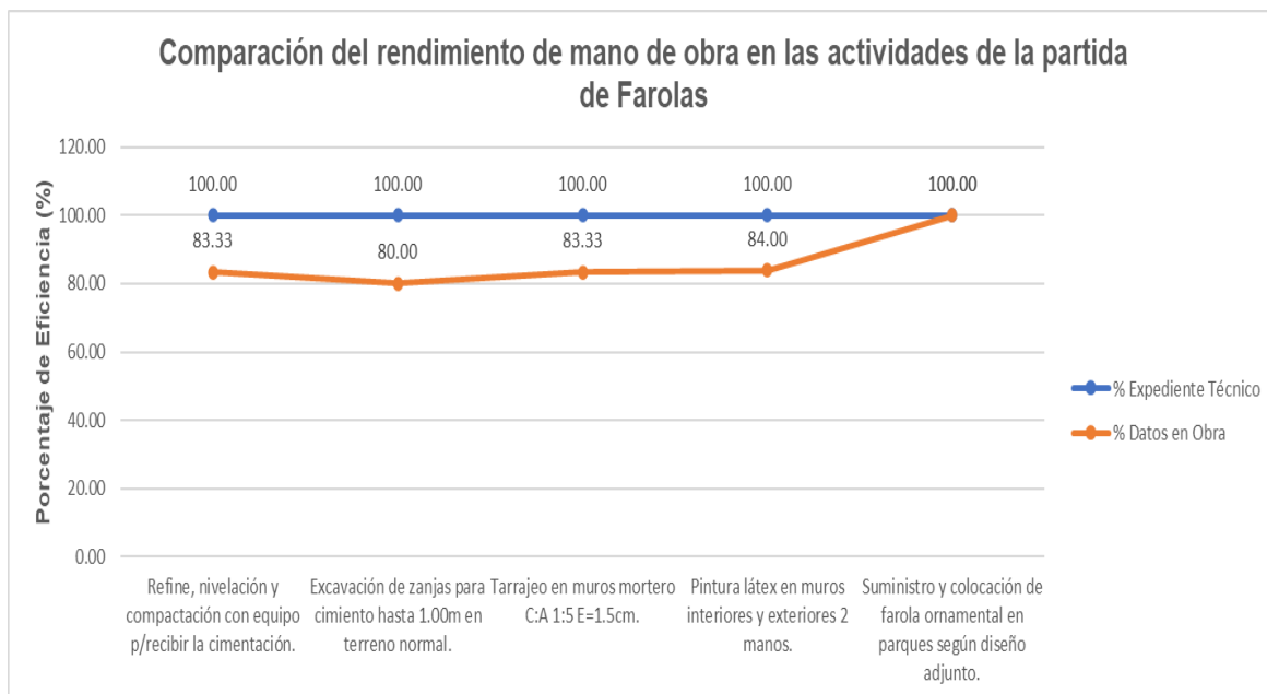
Figura 4. Comparación del rendimiento de mano de obra en las actividades de la partida de “farolas”.
