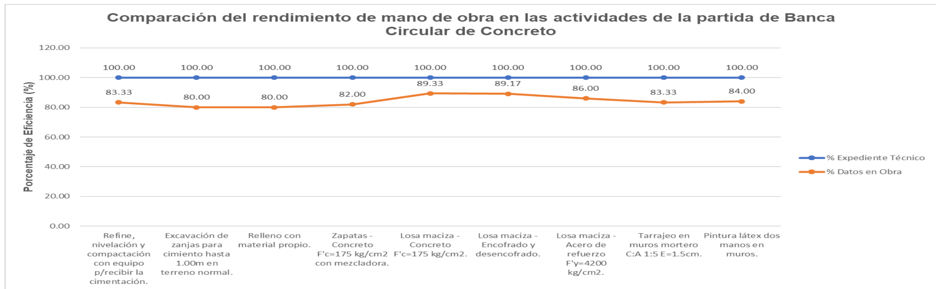
Figura 6. Comparación del rendimiento de mano de obra en las actividades de la partida de “banca circular de concreto”.
