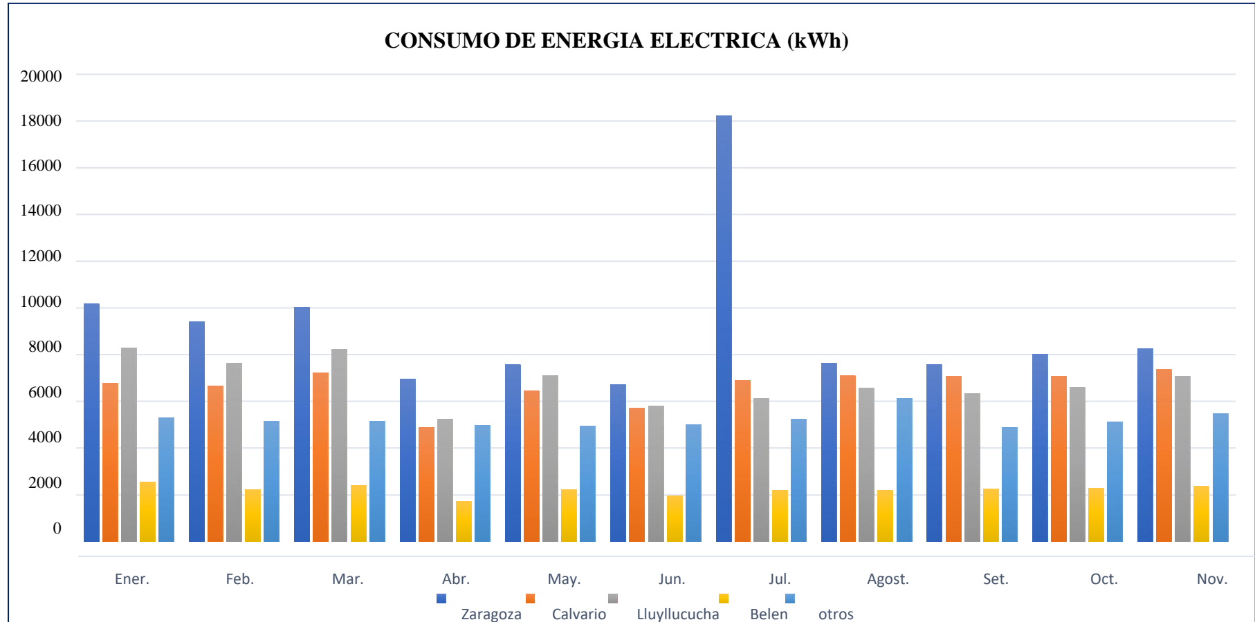
Figura 11. Resumen general del consumo total de electricidad (kWh).
