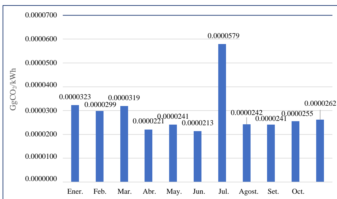
Figura 18. Carbono equivalente promedio (CO 2 eq) en el barrio Zaragosa.
