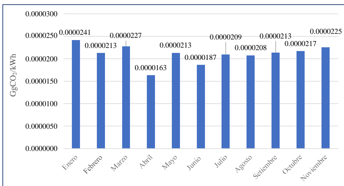
Figura 24. Carbono equivalente promedio ( \text{CO}_2 eq) en el barrio Belén.
