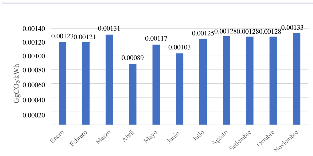
Figura 19. Carbono equivalente total ( \text{CO}_2 eq) en el barrio Calvario.
