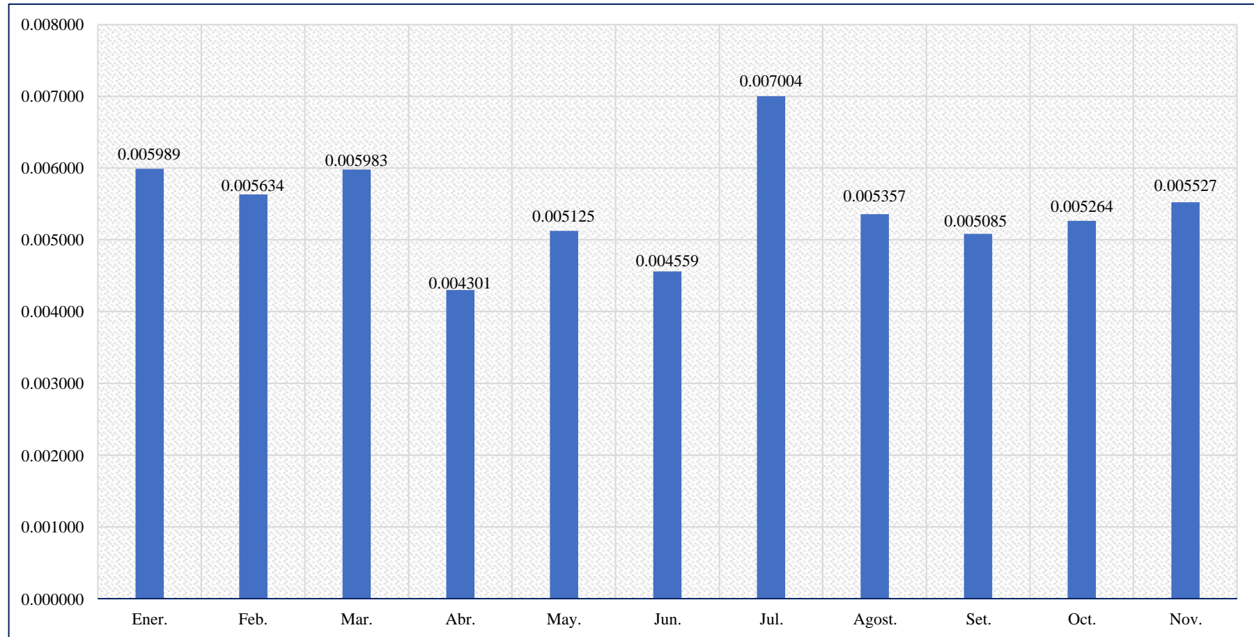
Figura 31. Resumen general de carbono equivalente total (CO 2 eq) generado por cada mes en Moyobamba.
