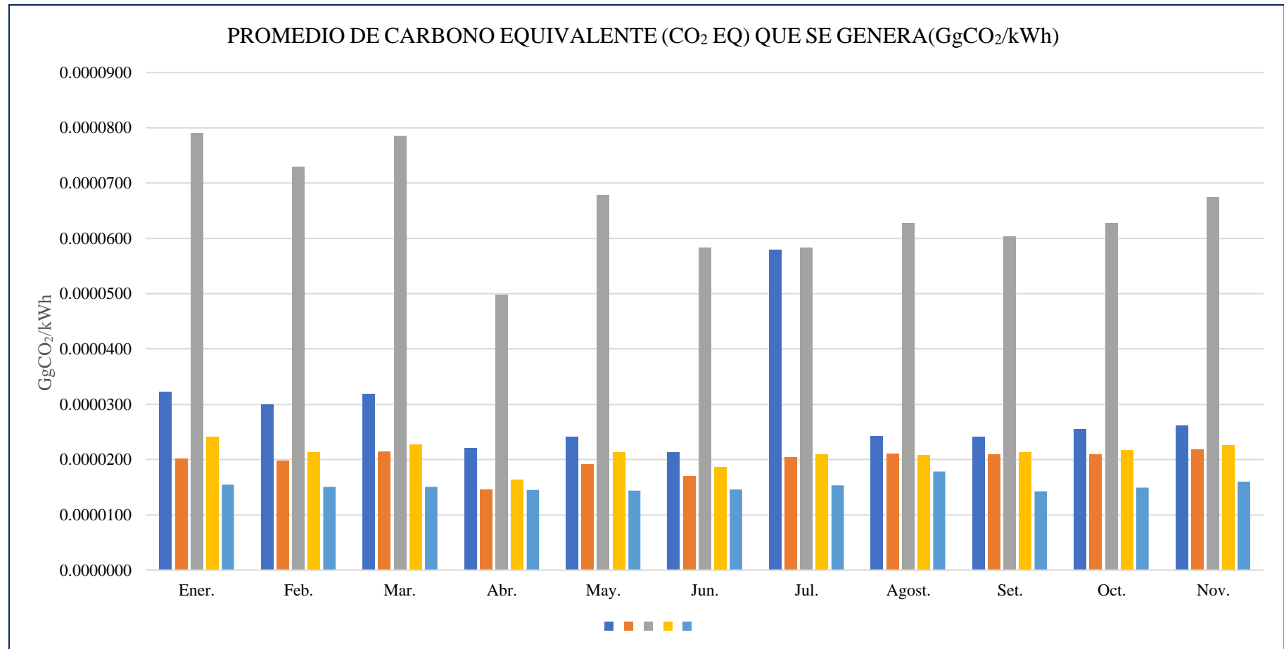
Figura 28. Resumen general de generación de carbono equivalente promedio (CO 2 eq).
