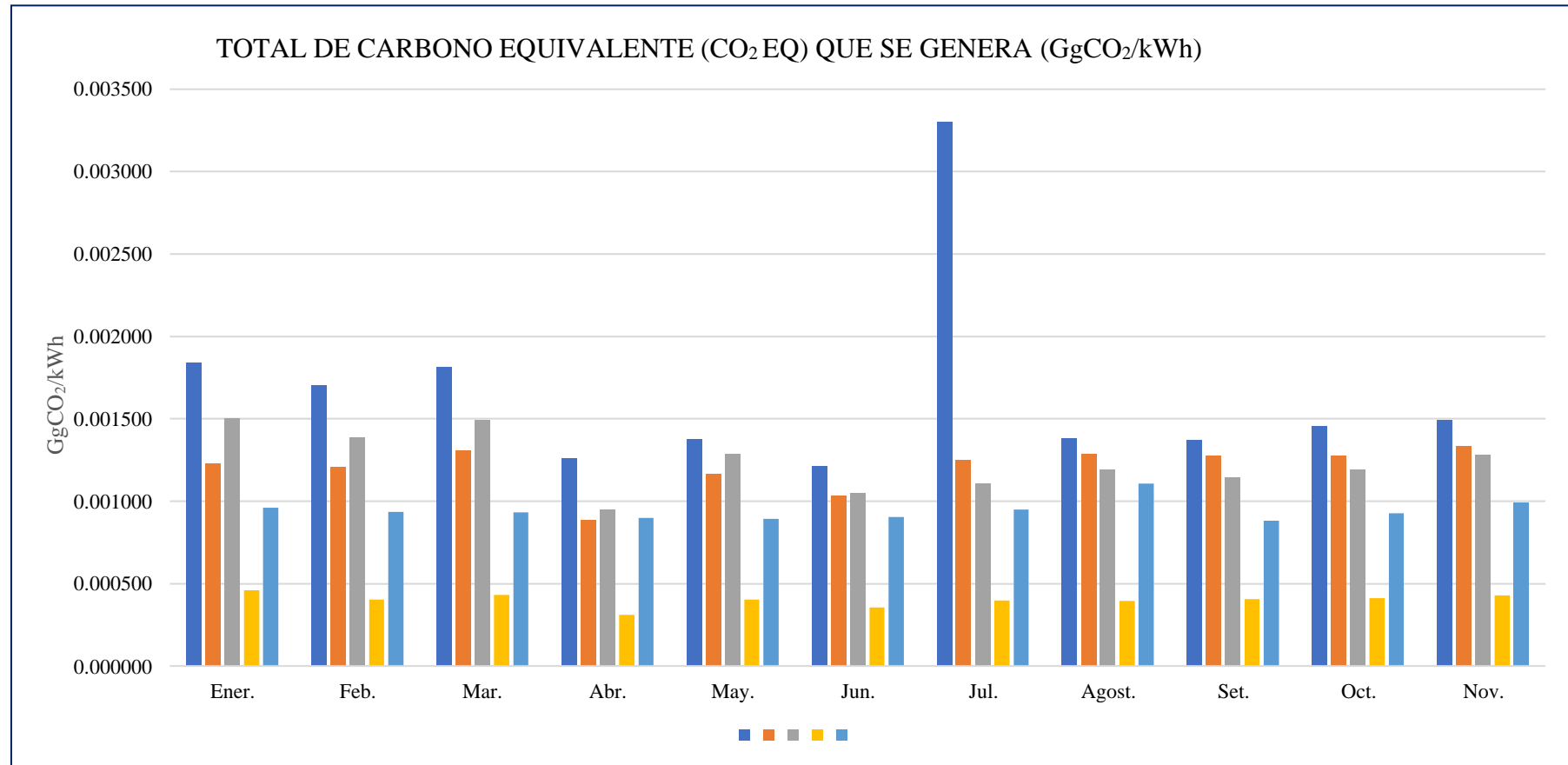
Figura 27. Resumen general de generación de carbono equivalente (CO 2 eq).
