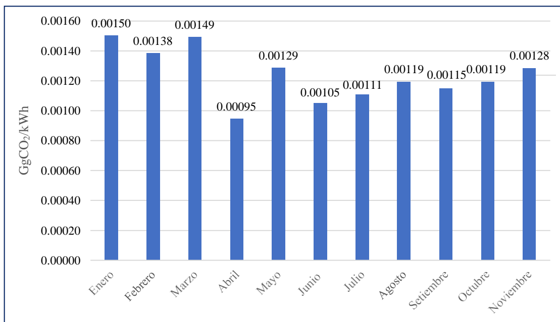
Figura 21. Carbono equivalente total ( \text{CO}_2 eq) en el barrio Lluylucucha.
