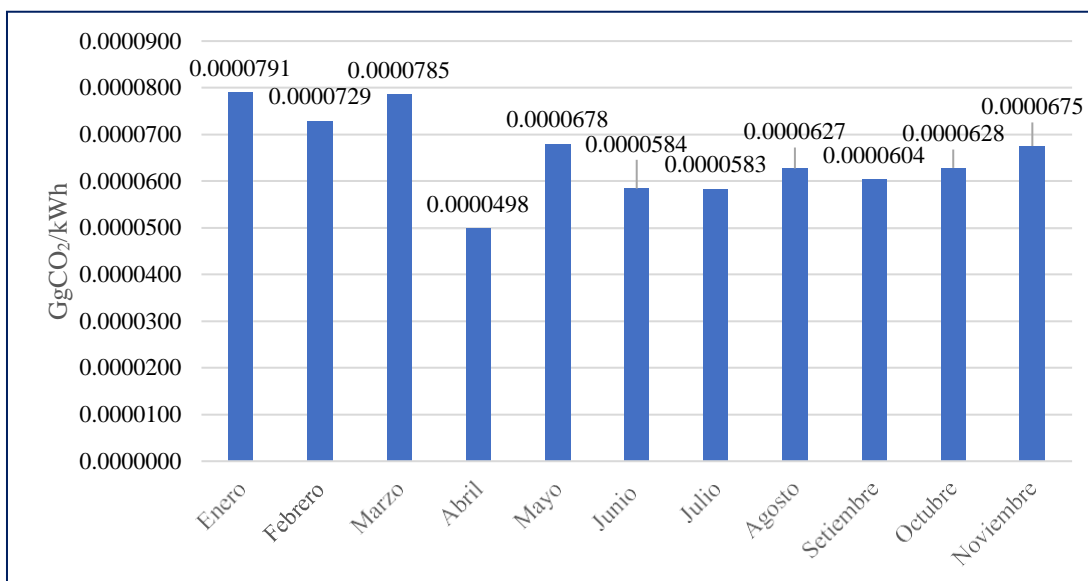
Figura 22. Carbono equivalente promedio ( \text{CO}_2 eq) en el barrio Lluylucucha.
