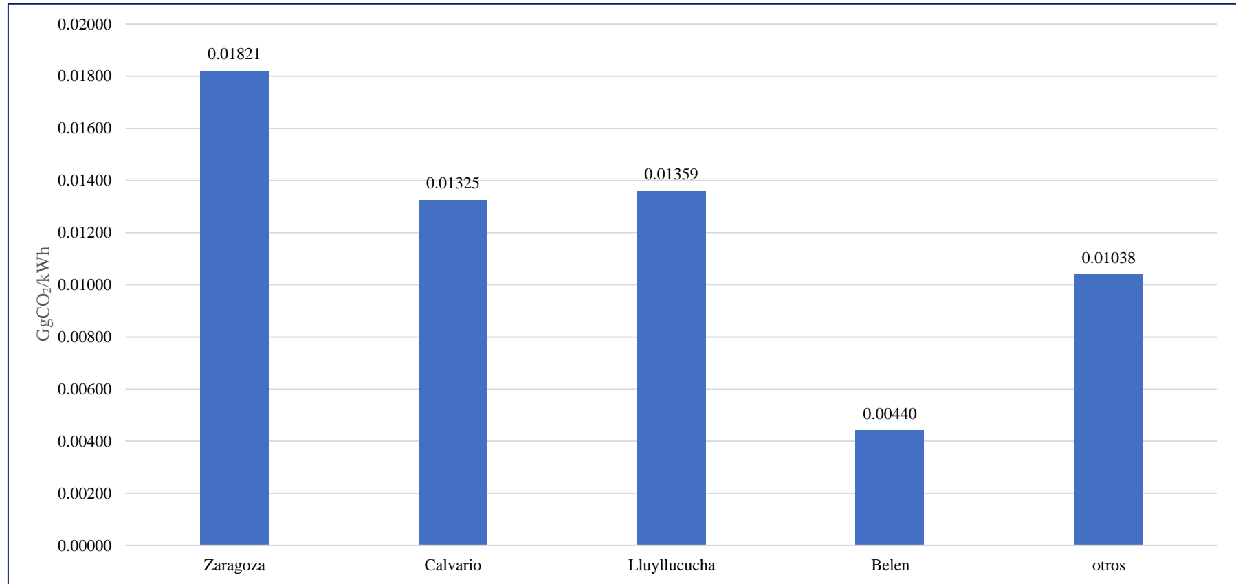
Figura 29. Resumen general de carbono equivalente (CO 2 eq) generado por cada barrio.
