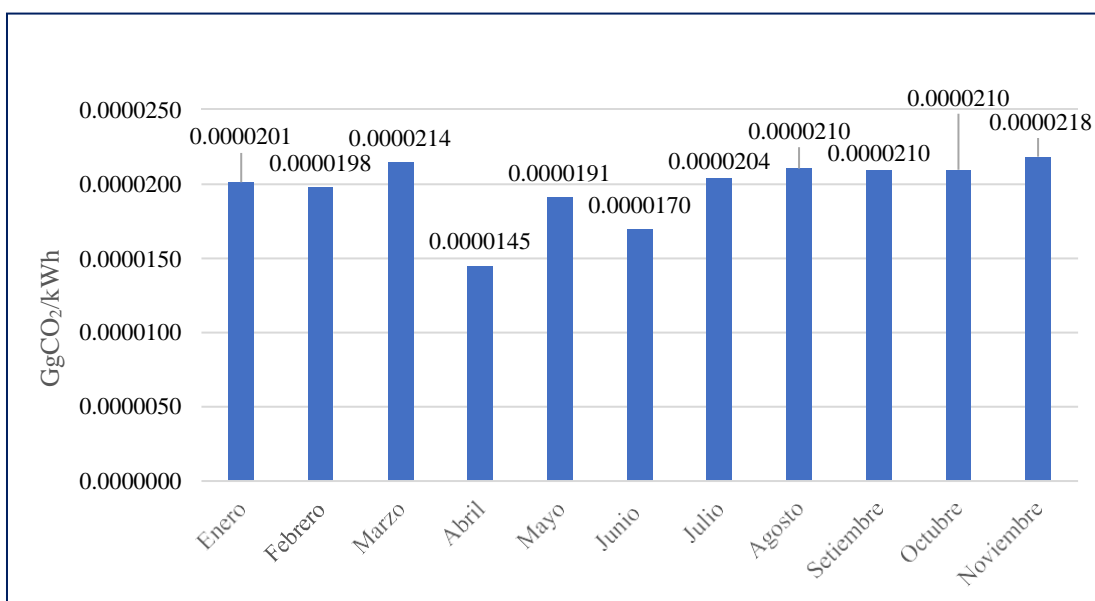
Figura 20. Carbono equivalente promedio ( \text{CO}_2 eq) en el barrio Calvario.
