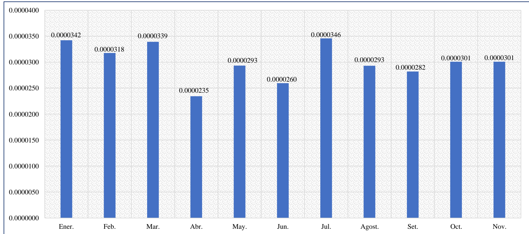
Figura 32. Resumen general de carbono equivalente promedio (CO 2 eq) generado por cada mes en Moyobamba.
