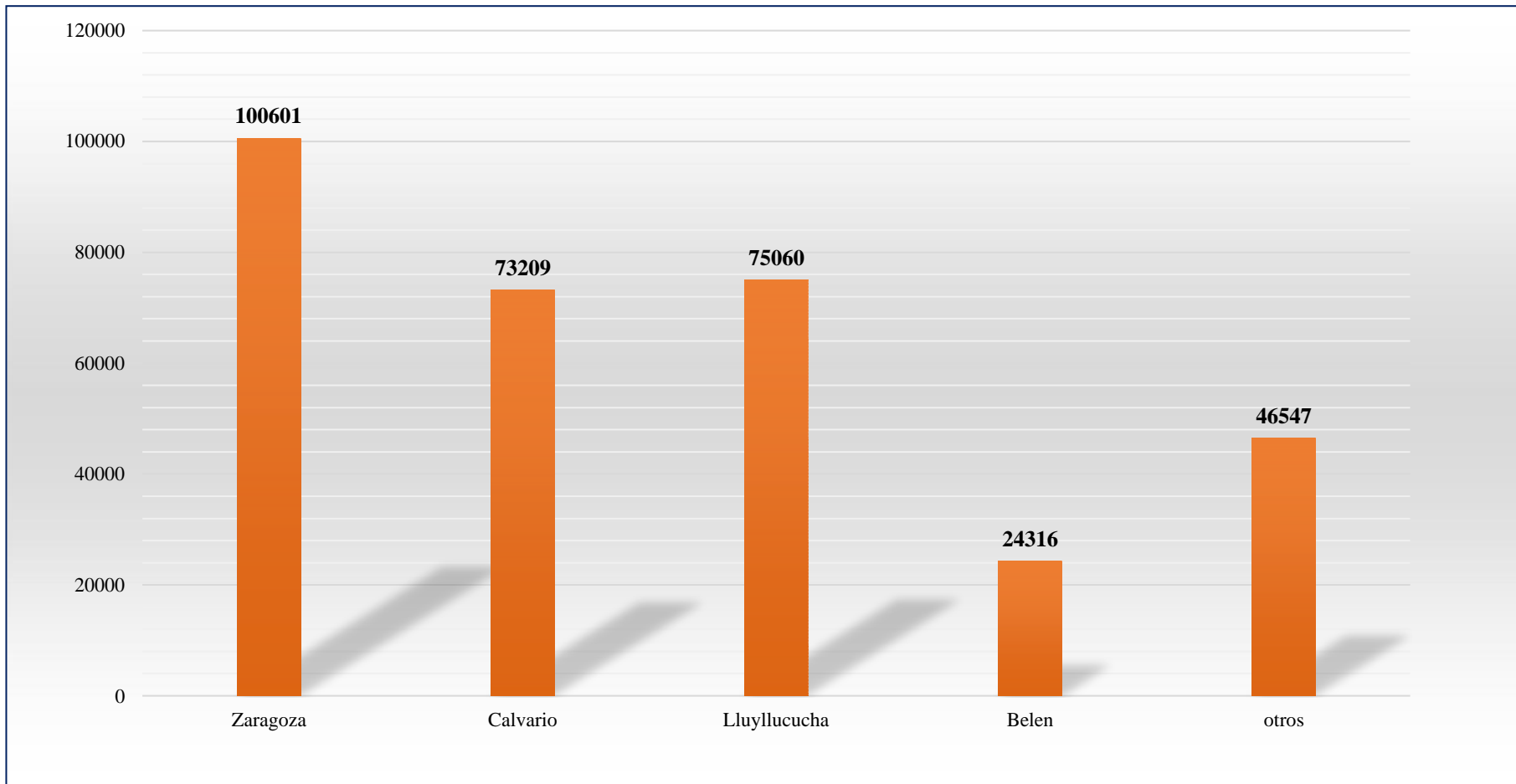
Figura 13. Resumen general del consumo de electricidad (kWh) por barrios.
