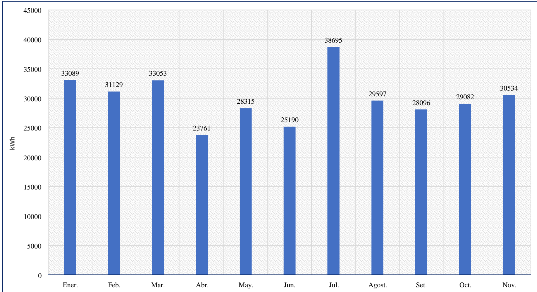
Figura 15. Resumen general del consumo total por mes de electricidad (kWh) en Moyobamba.
