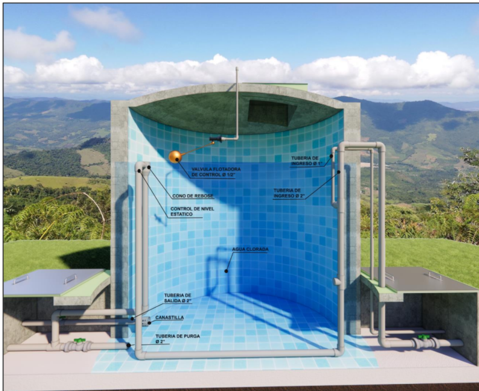
Figura 4 Instalación del nivel estático
