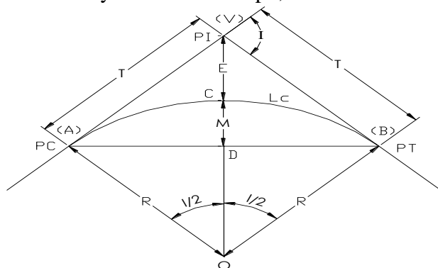
ELEMENTOS DE UNA CURVA SIMPLE
