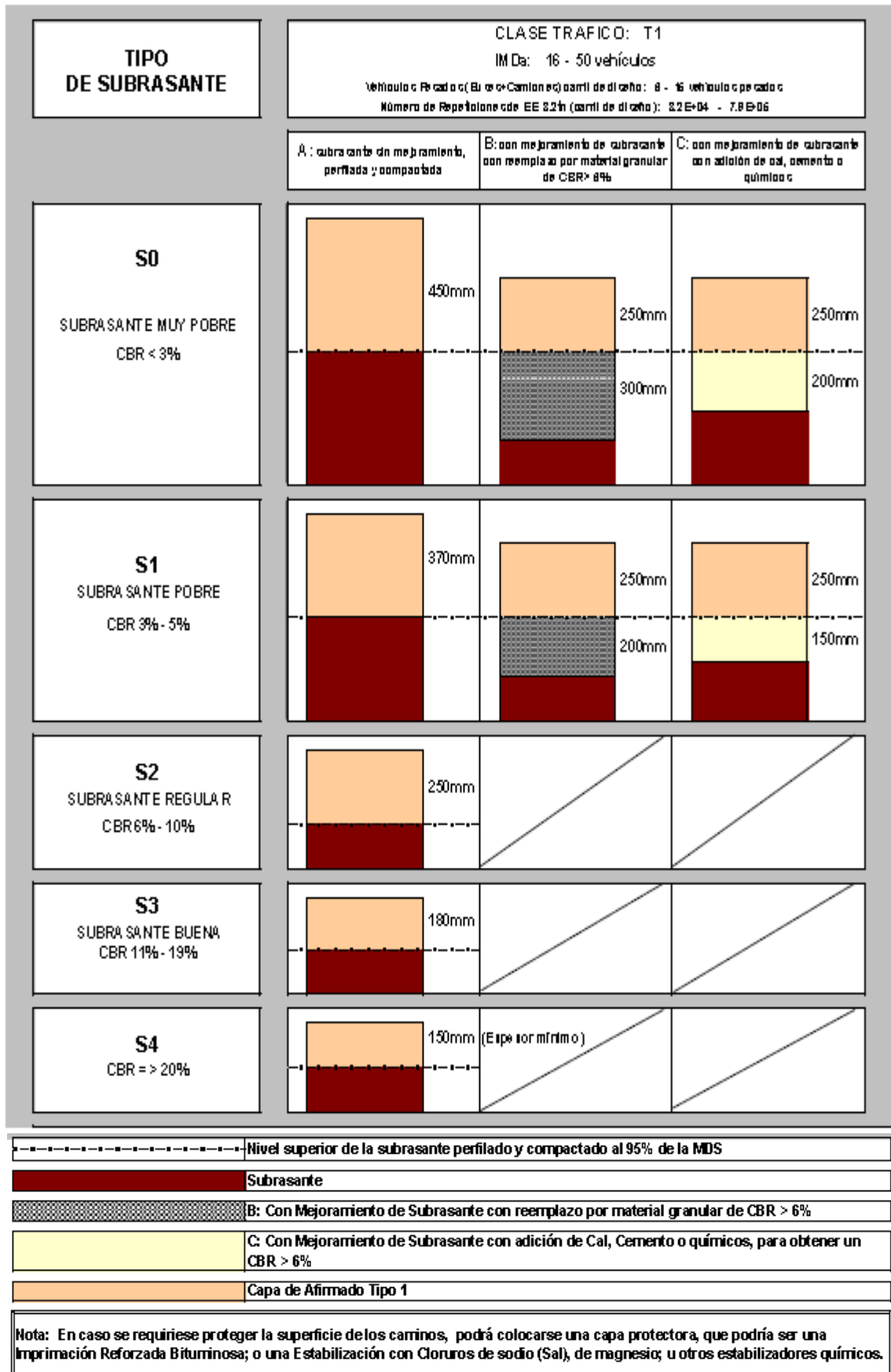
Figura 7. Catálogo de Capas de Revestimiento Granular (fuente: ministerio de transportes y comunicaciones)
