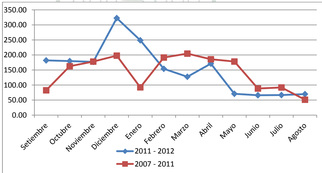
Gráfico N° 03: Variación de la Precipitación Total mes (mm) en los años 2007 -2011(Patrón Histórico) y 2011-2012 (Estudio) Setiembre-Agosto, registrado por SENAMHI.
