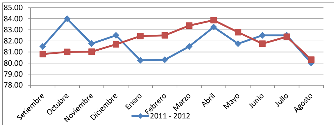
Gráfico N° 02: Variación de la Humedad Relativa en los años 2007 - 2011(Patrón Histórico) y 2011-2012 (Estudio) Setiembre-Agosto, registrado por SENAMHI.
