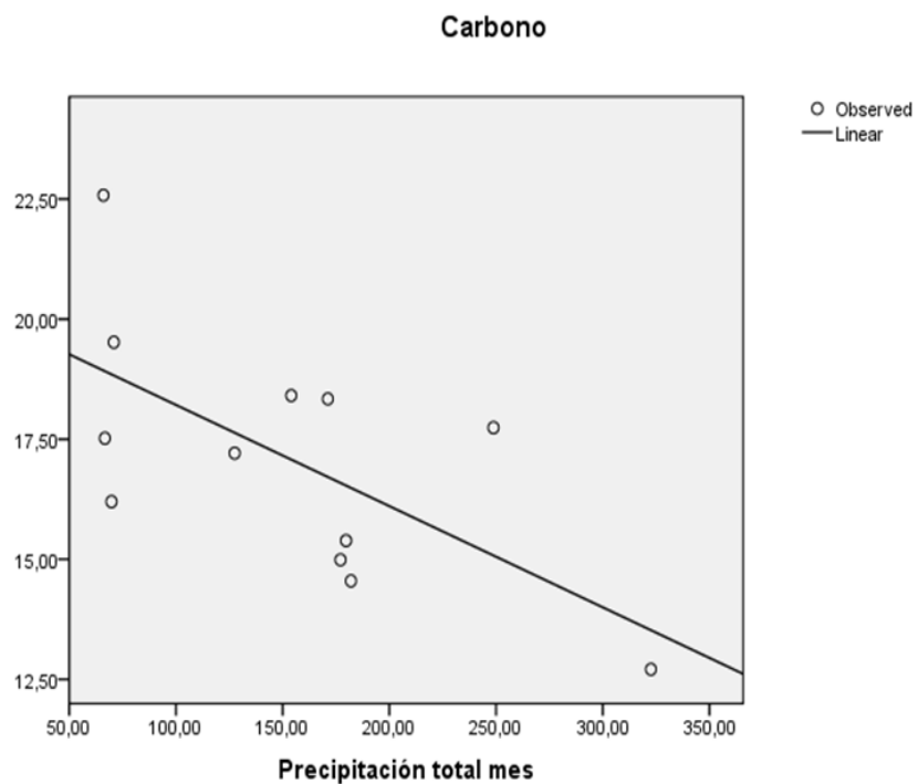
Gráfico N° 09: Diagrama de dispersión de la captura de carbono y precipitación en la Comunidad alto el sol, Pachiza 2012.
