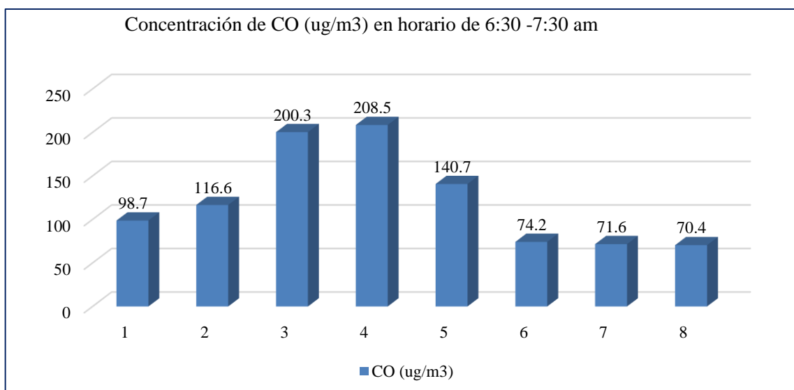
Figura 27. Concentración de CO (ug/m 3 ) – horario mañana.
