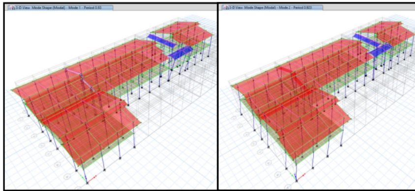
Figura 26. Periodo fundamental en la dirección "X" e "Y" - Pabellón de Laboratorios y Gabinetes de la Facultad de Ciencias Agrarias
