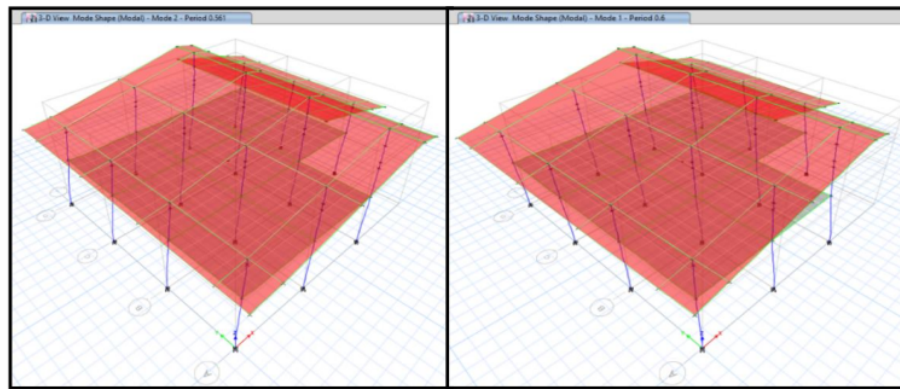
Figura 29. Periodo fundamental en la dirección "X" e "Y" - Pabellón de Administrativo 01 de ambas Facultades de Ciencias Agrarias e Ingeniería Agroindustrial
