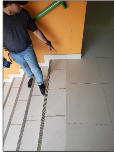
Foto N° 14: Presencia de fisuras en las paredes justo en los de bloques de la escalera de acceso y los ambientes de Administrativo 02 donde no existe junta de separación de la Facultad de Ingeniería Agroindustrial (Fuente: Elaboración propia)
