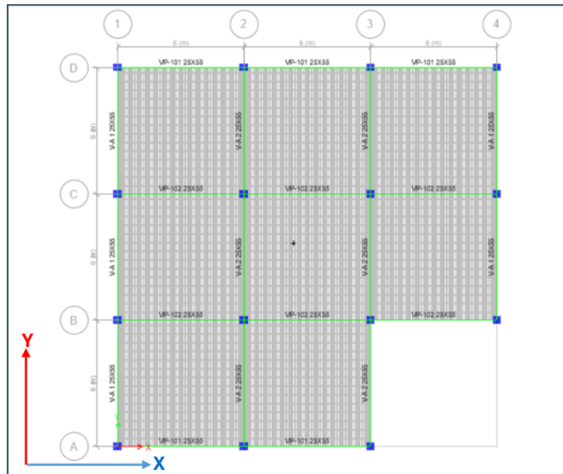
Figura 19. Sistemas de ejes definidos tanto para la dirección X-X y Y-Y - Pabellón de Administrativo 01 para ambas Facultades de Ciencias Agrarias e Ingeniería Agroindustrial
