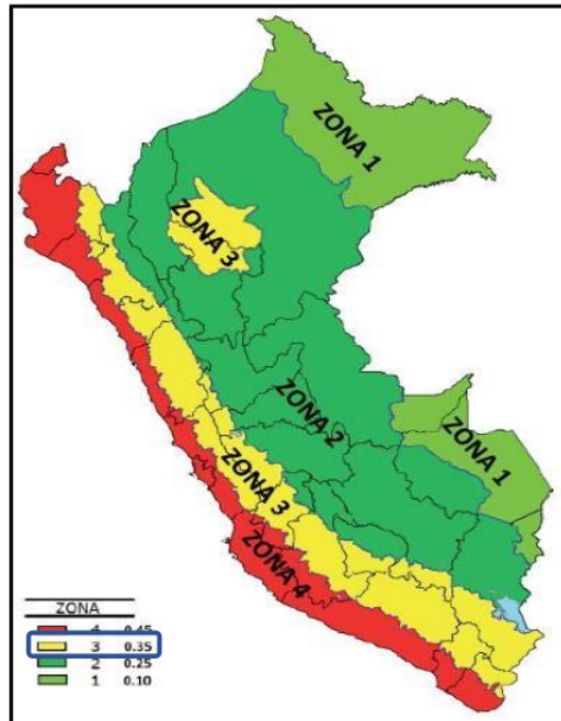
Figura 4. Factores de zona "Z" para cada zona sísmica
