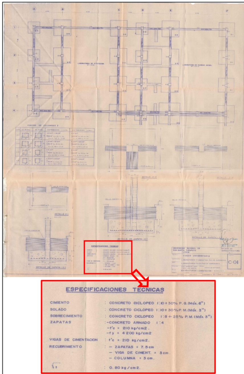
Figura 3. Especificaciones técnicas y capacidad portante del suelo, tomadas de los planos de estructuras del Pabellón de Laboratorios y Gabinetes de la Facultad de Ciencias Agrarias
