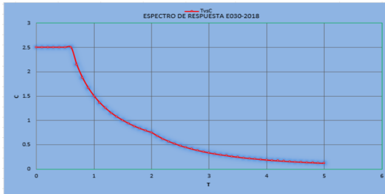
Figura 24. Gráfico del Espectro Pseudoaceleraciones "T" vs "C"
