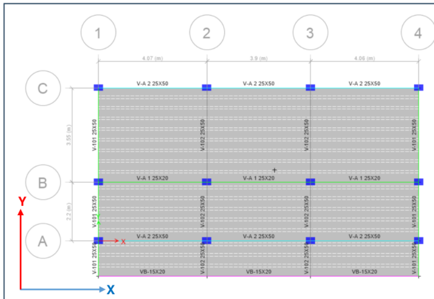
Figura 17. Sistemas de ejes definidos tanto para la dirección X-X y Y-Y - Pabellón de SS-HH para ambas Facultades de Ciencias Agrarias e Ingeniería Agroindustrial
