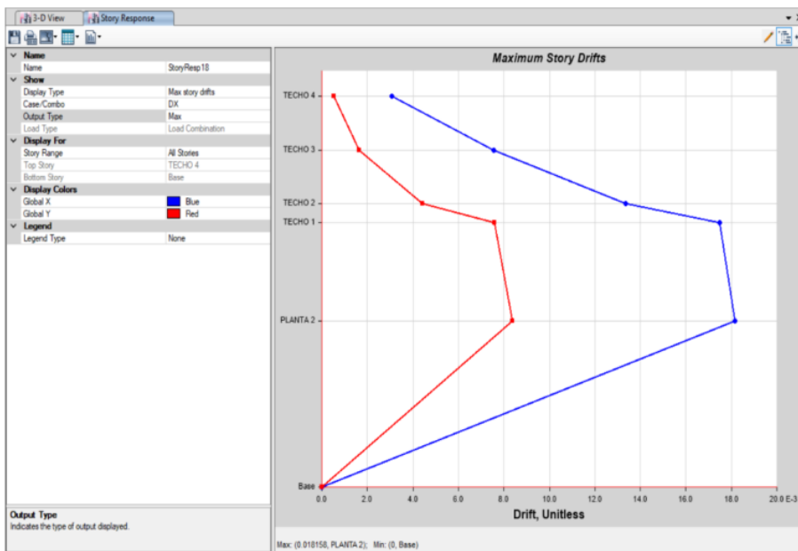
Figura 41. Distorsiones máximas en la Dirección X-X - Pabellón de Administrativo 02 de ambas Facultades de Ciencias Agrarias e Ingeniería Agroindustrial
