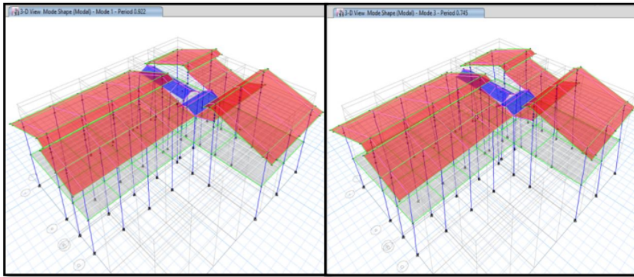
Figura 27. Periodo fundamental en la dirección "X" e "Y" - Pabellón de Laboratorios de la Facultad de Ingeniería Agroindustrial
