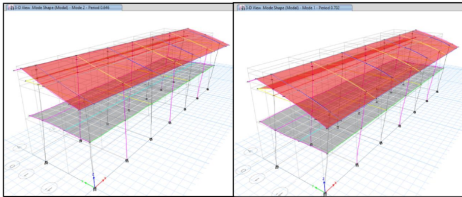
Figura 25. Periodo fundamental en la dirección “X” e “Y” - Pabellón de Aulas de ambas Facultades de Ciencias Agrarias e Ingeniería Agroindustrial
