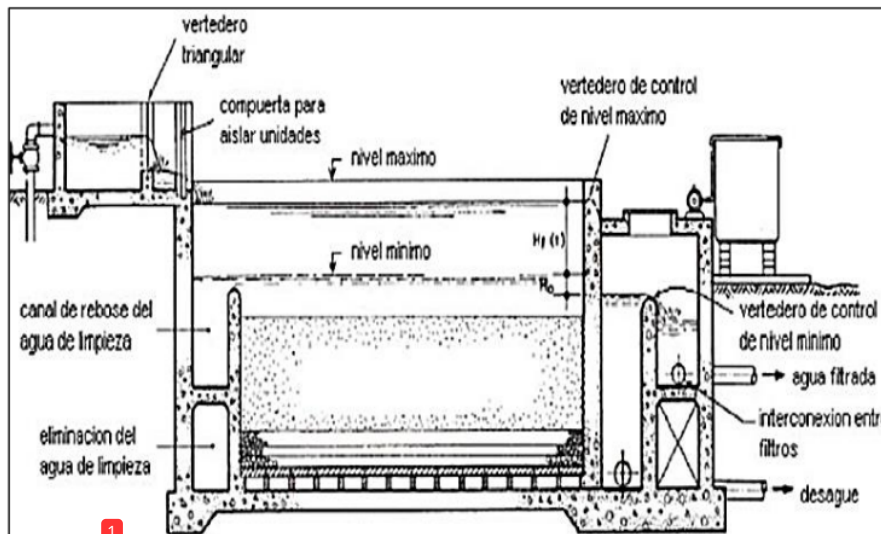
Figura 8. Corte longitudinal de un filtro lento de arena.
