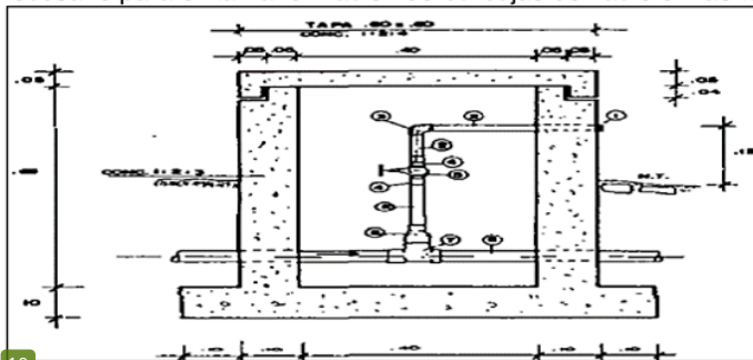
Figura 2. Válvula de aire manual.
