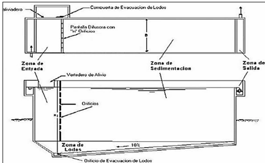
Figura 7. Sedimentador-Planta y corte longitudinal.
