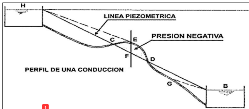
Figura 10. Perfil de presión negativa.
