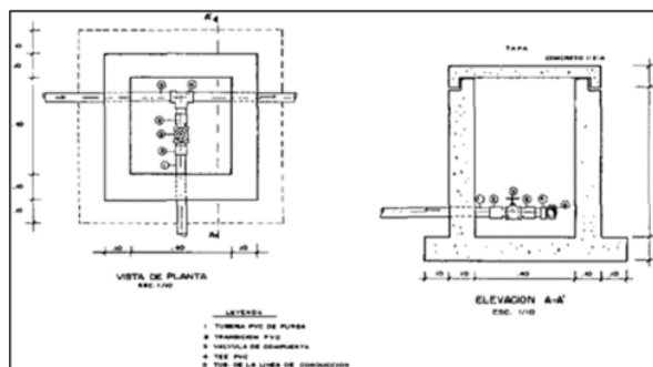
Figura 3. Válvula de purga.
