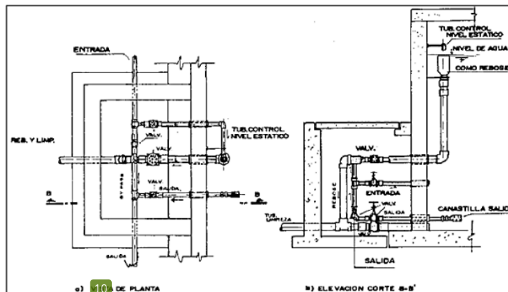
Figura 6. Caseta de válvulas de reservorio.
