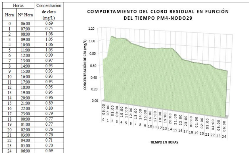
Figura 19. Comportamiento del Cloro Residual en función del tiempo PM4 - Nodo 29.
