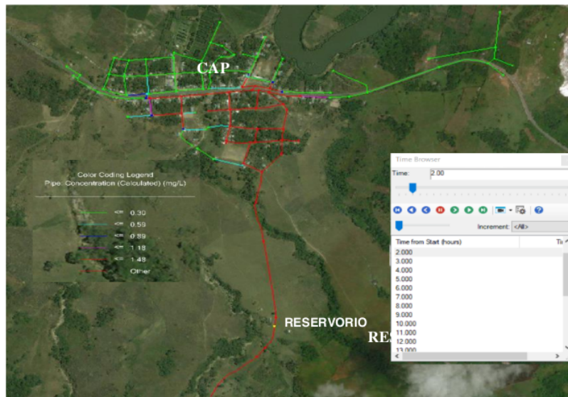
Figura 13. Concentración de cloro en redes de distribución.
