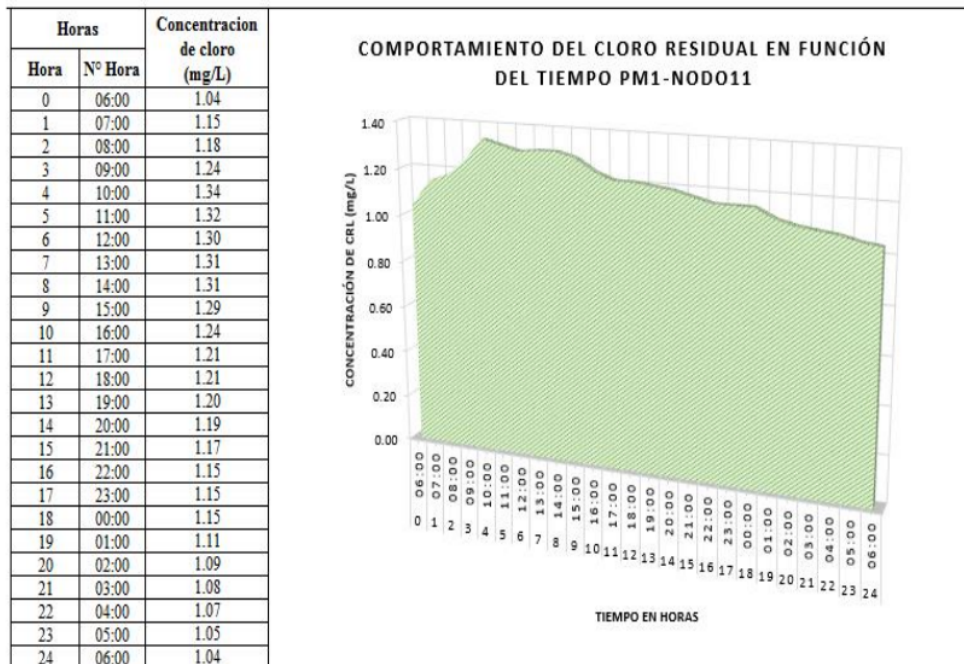
Figura 16. Comportamiento del Cloro Residual en función del tiempo PM1 - Nodo 11.
