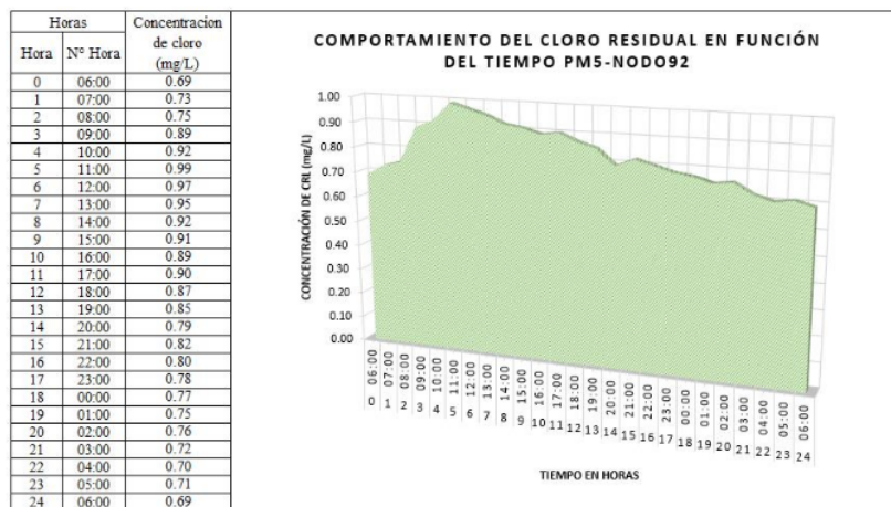
Figura 20. Comportamiento del Cloro Residual en función del tiempo PM5 - Nodo 92 Interpretación
