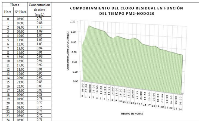
Figura 17. Comportamiento del Cloro Residual en función del tiempo PM2 - Nodo 20
