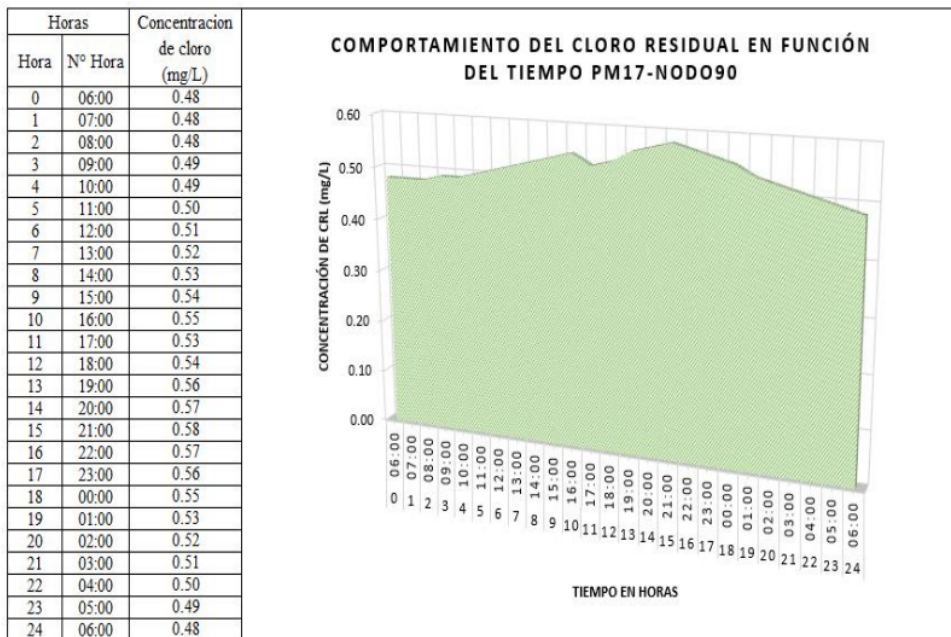
2 Figura 32. Comportamiento del Cloro Residual en función del tiempo PM17 - Nodo 90
