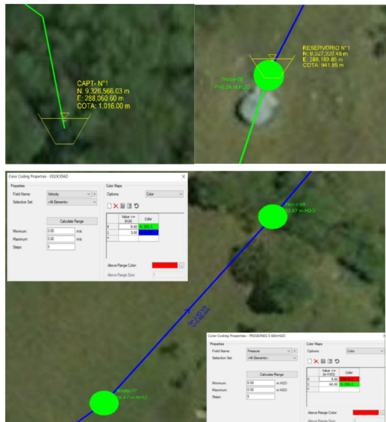
Figura 8. Simulación hidráulica del sistema de distribución de agua en el C.P. Marona.
