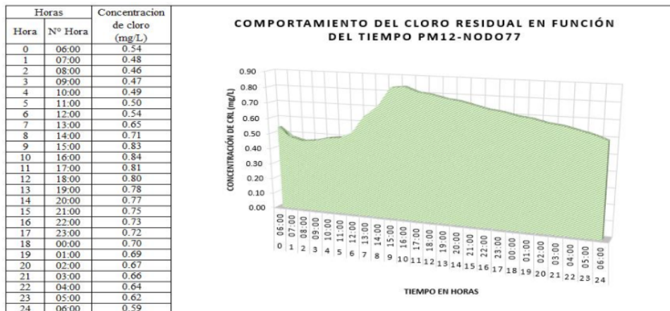
Figura 27. Comportamiento del Cloro Residual en función del tiempo PM12 - Nodo 77
