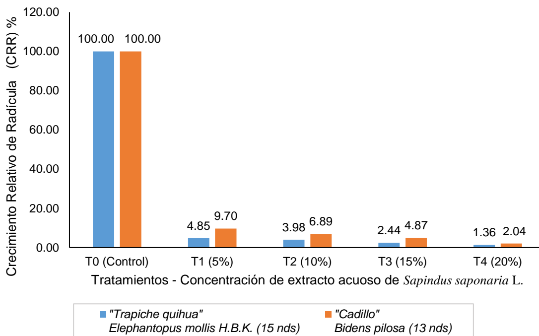
Figura 6. Crecimiento Relativo de Radícula (CRR), según concentración de extracto acuoso del mesocarpio del fruto de Sapindus saponaria L. en semillas de malezas aceptoras (bionesayo); (nds): Número de días después de la siembra.
