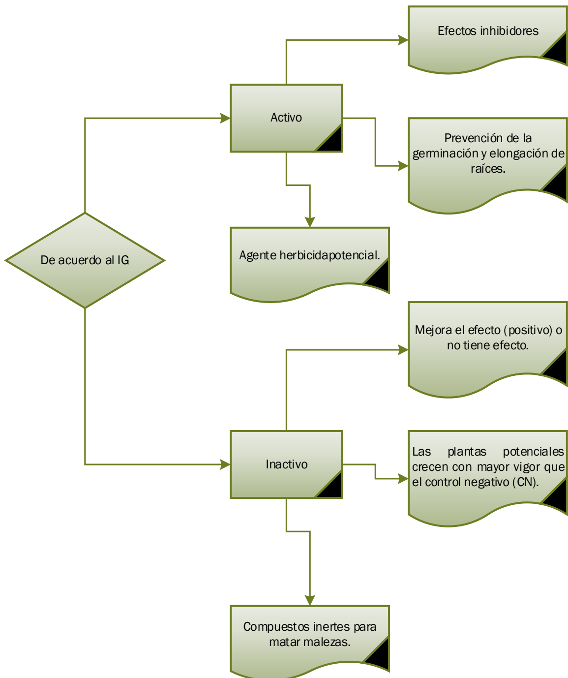
Figura 4. Criterios para la selección de los extractos activos e inactivos
