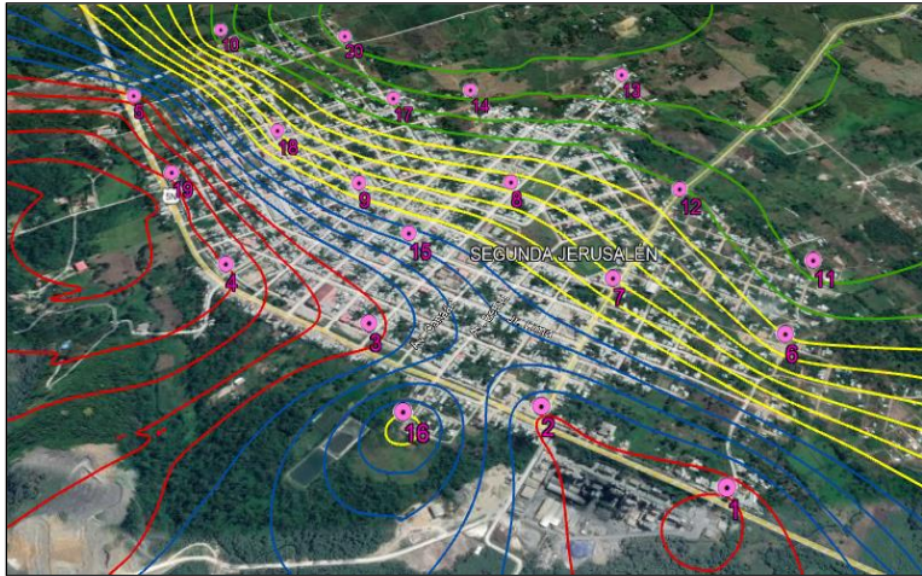
Figura 7. Representación geo espacial del comportamiento del ruido en la localidad de Segunda Jerusalén.
