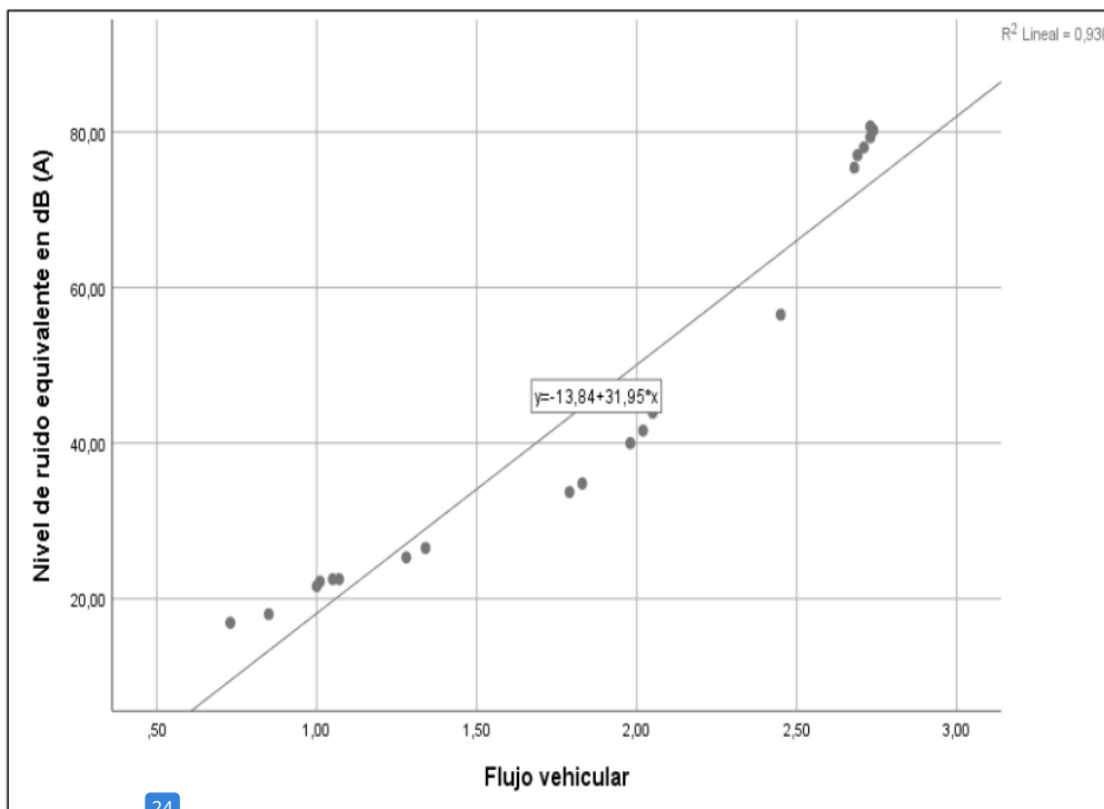
24 Figura 5. Modelo de regresión lineal en horario de la tarde en la ciudad de Segunda Jerusalén.
