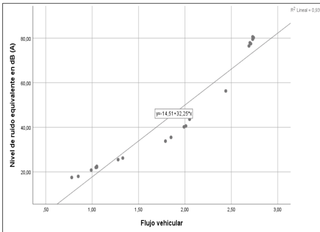
Figura 6. Modelo de regresión lineal diario en la ciudad de Segunda Jerusalén.
