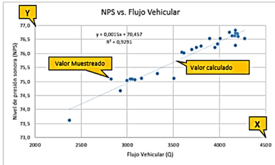
Figura 1. Regresión lineal
