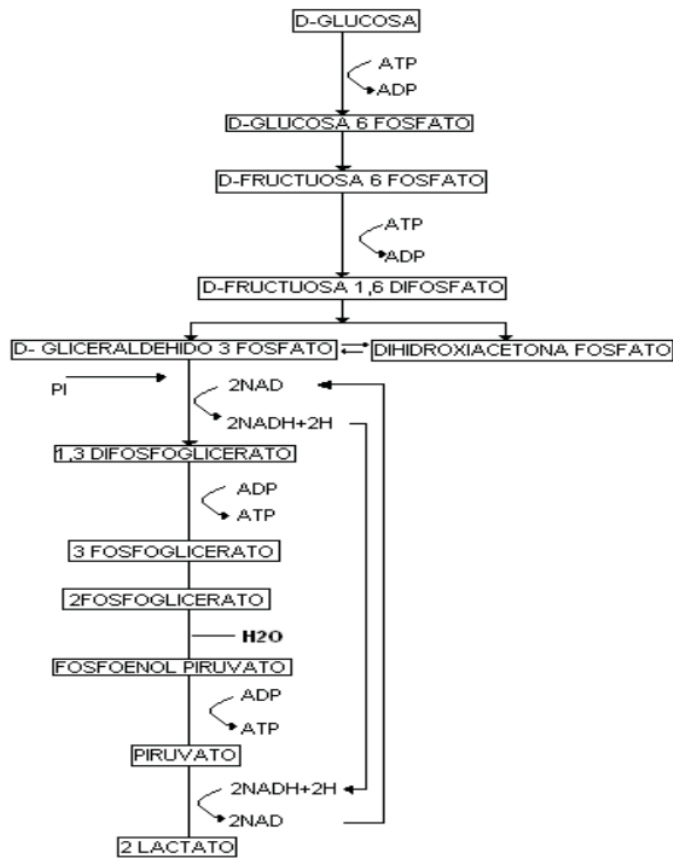
Figura 1. Fermentación homoláctica
