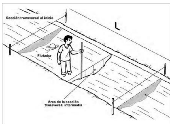
Figura 23. Medición con el método del correntómetro
