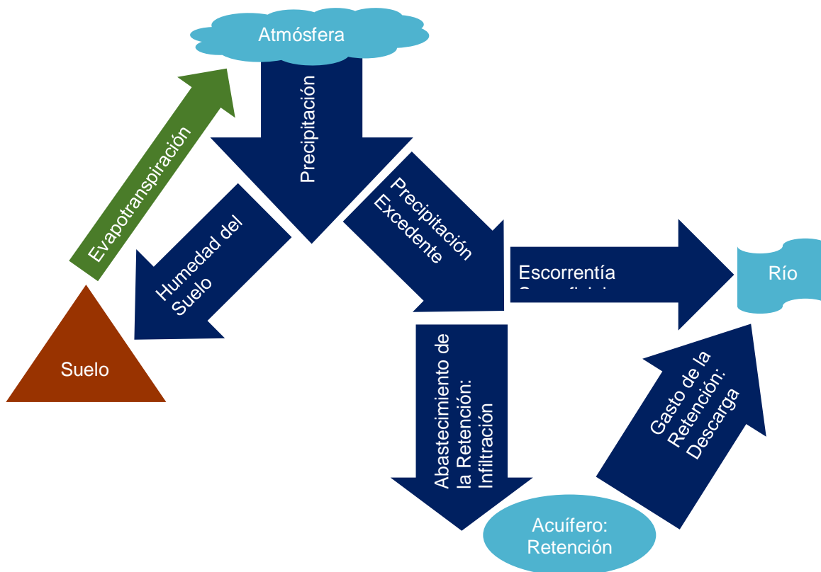
Figura 2. Flujo de la precipitación según ecuación del Balance Hídrico Fuente: Elaboración Propia (2019)
