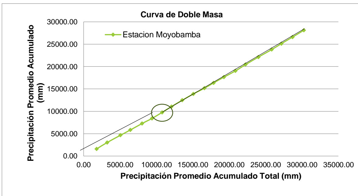
Figura 18. Curva de Doble Masa de la Estación Moyobamba Fuente: Elaboración propia
