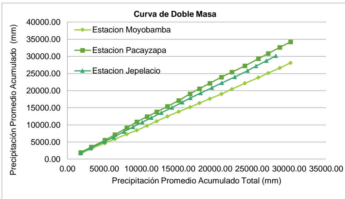
Figura 17. Curva de Doble Masa de las Estaciones consideradas en el estudio Fuente: Elaboración propia
