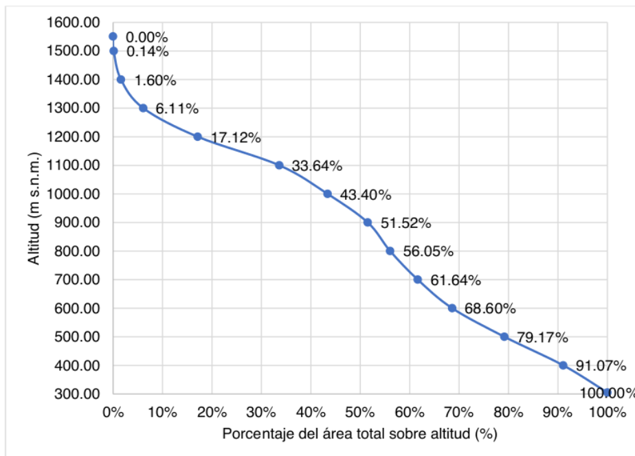
Figura 47. 1 Curva hipsométrica de la microcuenca de la quebrada Yuracyacu.
