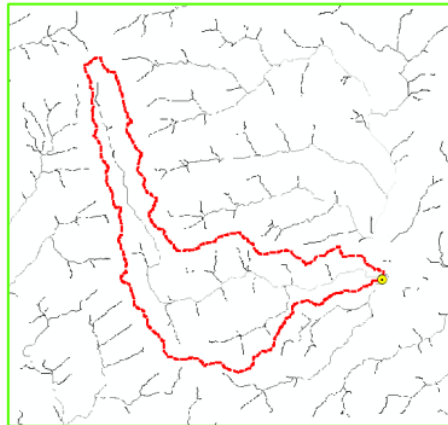
Figura 14. Densidad establecida para las líneas de escurrimiento.
