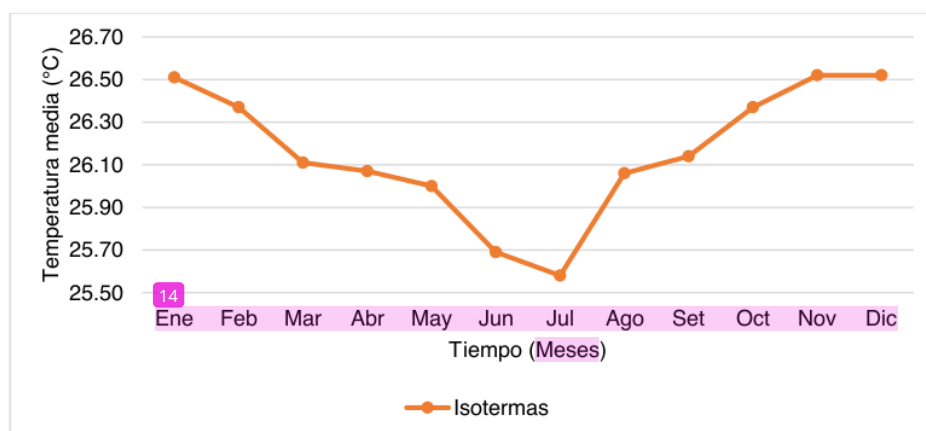
Figura 50. Temperatura media mensual de la microcuenca de la quebrada Yuracyacu.
