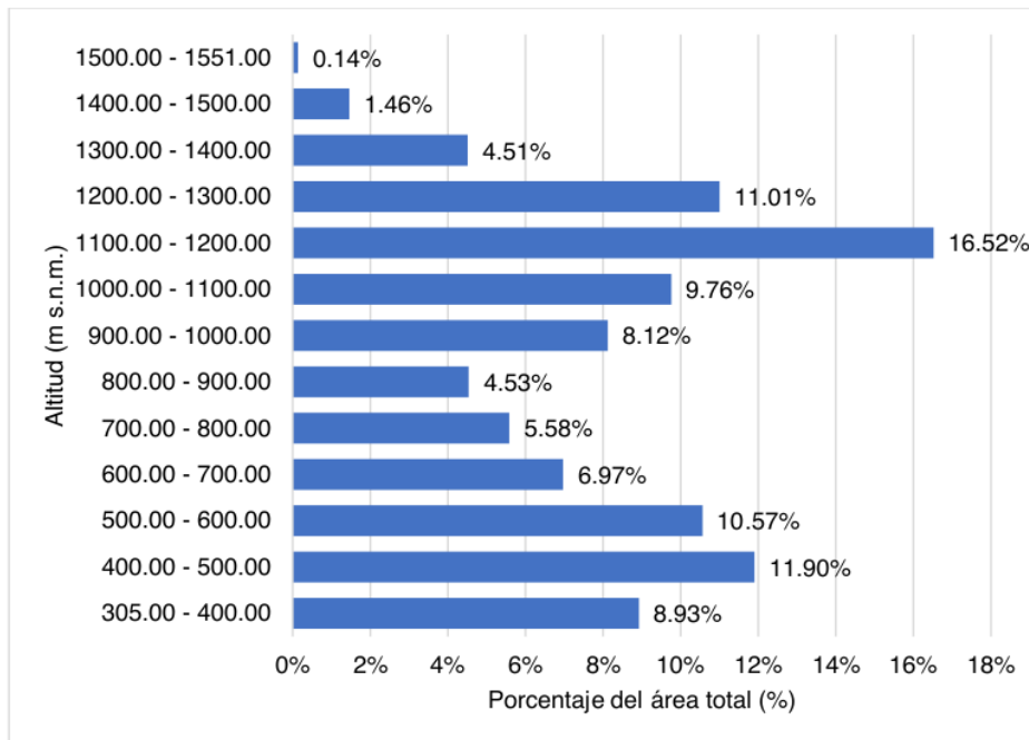
Figura 46. 2 Histograma de frecuencia de altitudes de la microcuenca de la quebrada Yuracyacu.
