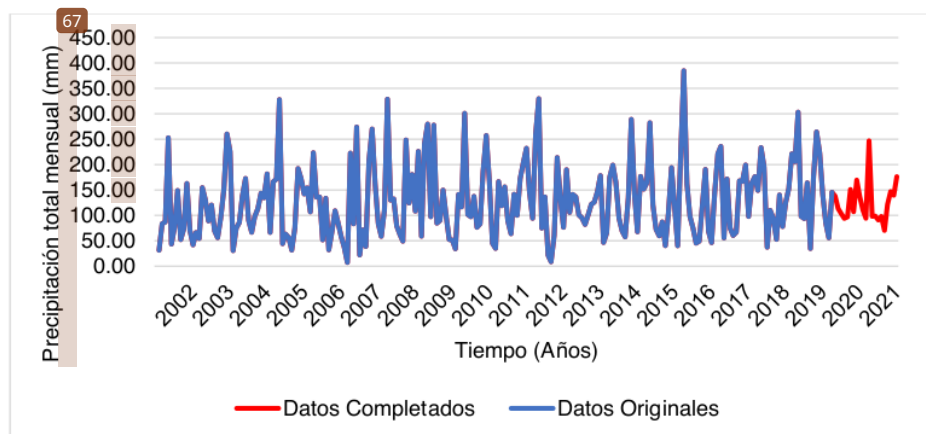
Figura 20. Análisis visual gráfico - Precipitación (Estación Alao).
