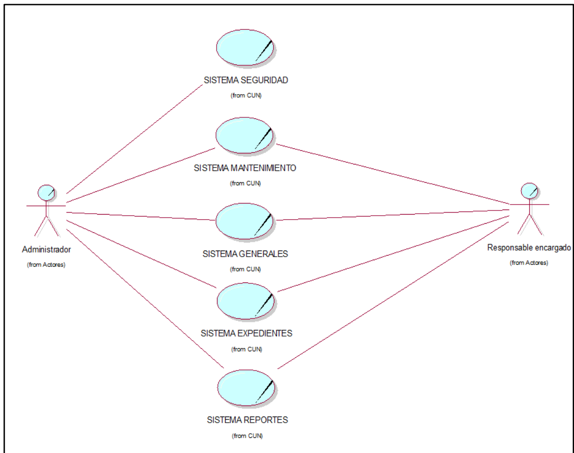
Figura 19 Diagrama de caso de uso
